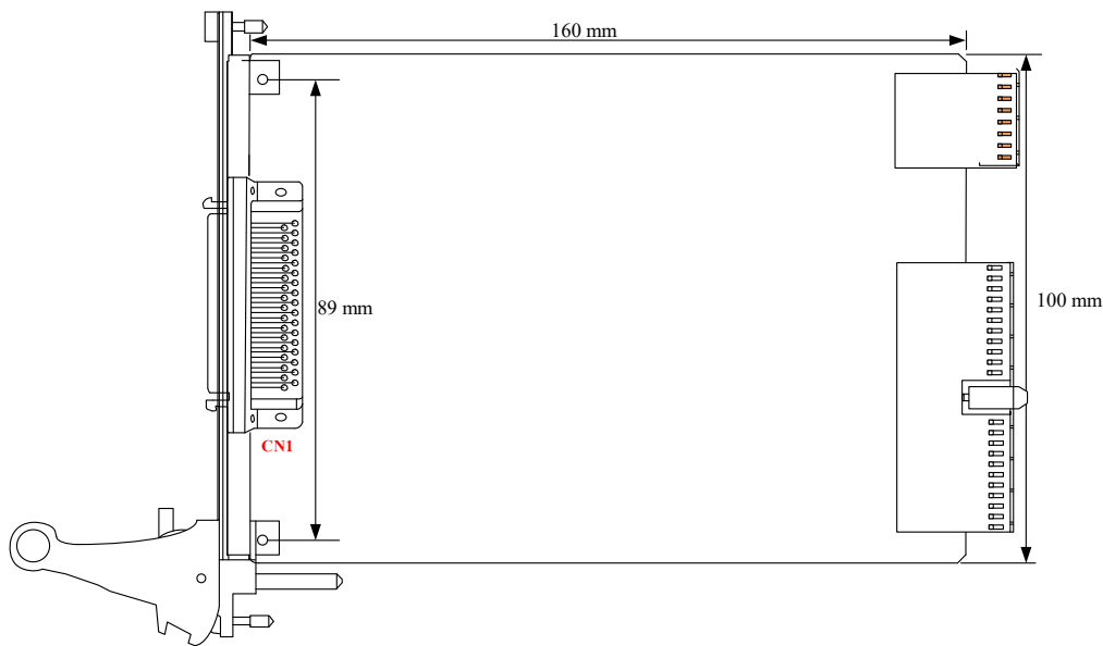
图 2-3-1 板卡尺寸图
