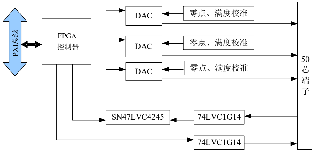
图 2-1-1 板卡原理框图
