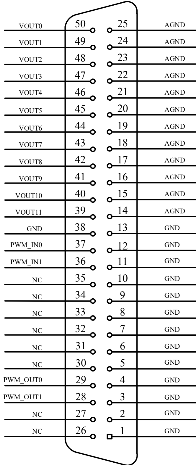
图 3-1-1 连接器定义图
