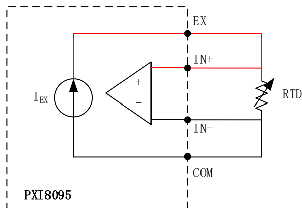
图 4-1-2 四线制测量
