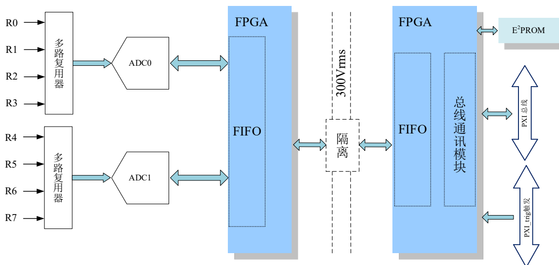
图 2-2-1 PXI8095 系统框图
