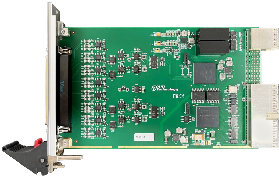
图 3-1-1 PXI8095 外形图
