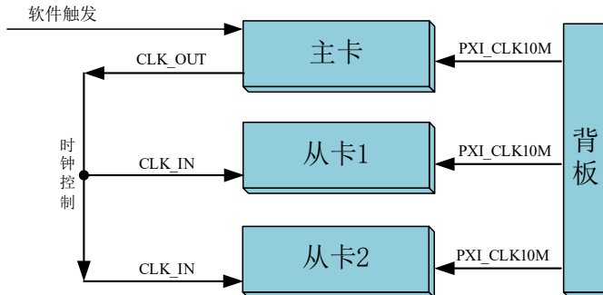
图 4-6-1 主从卡级联时钟同步
