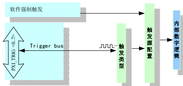
图 4-5-1 AI 触发功能框图
