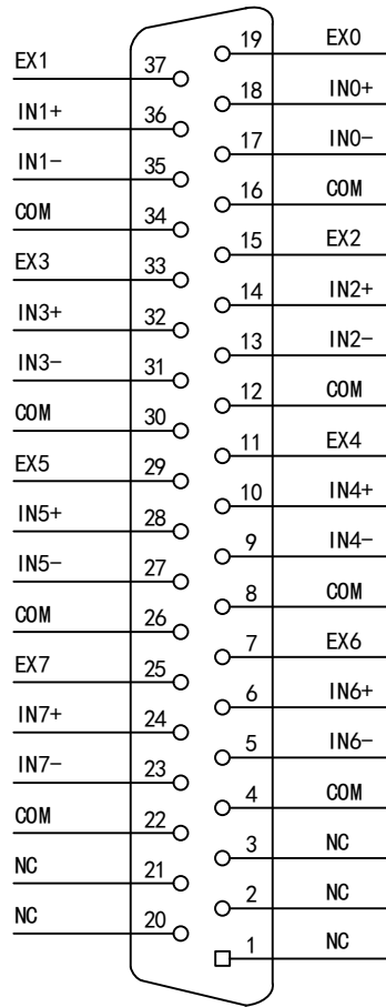
图 3-3-2 PXI8095 端子引脚定义
