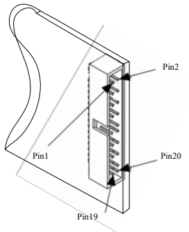
图 3-3-2 RTSI 的 Pinout 图
