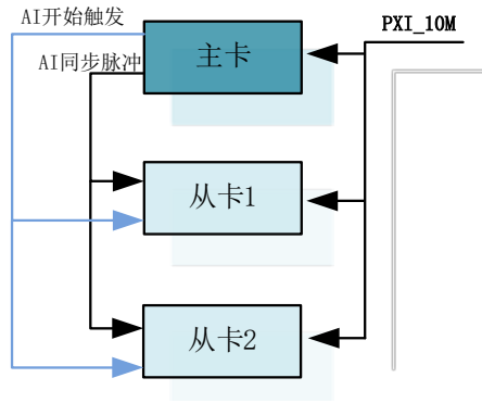
图 4-10-1 主从卡级联
