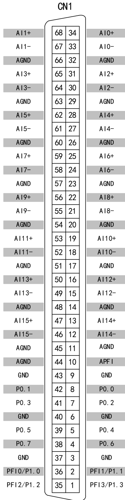
图 3-3-1 2880/A/B 管脚定义图
