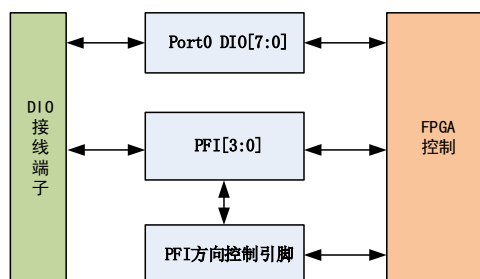
图6-1-1 DIO功能框图
