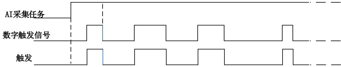
图7-3-7 数字边沿触发--下降沿触发
