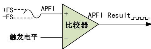
图7-3-4 模拟触发比较器
