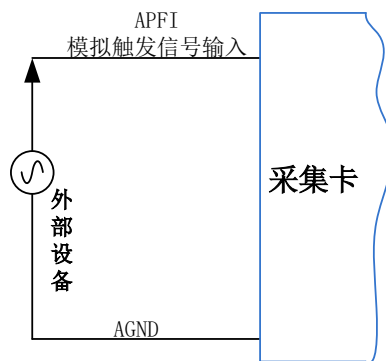
图7-3-3 模拟触发连接方法
