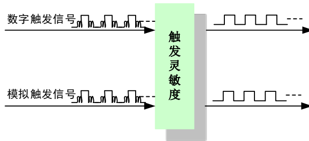
图 7-3-1 触发灵敏度
