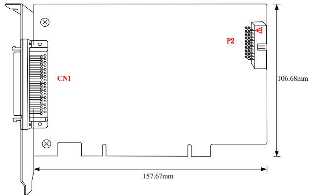
图 3-2-1 PCI2880/A/B 板卡尺寸图
