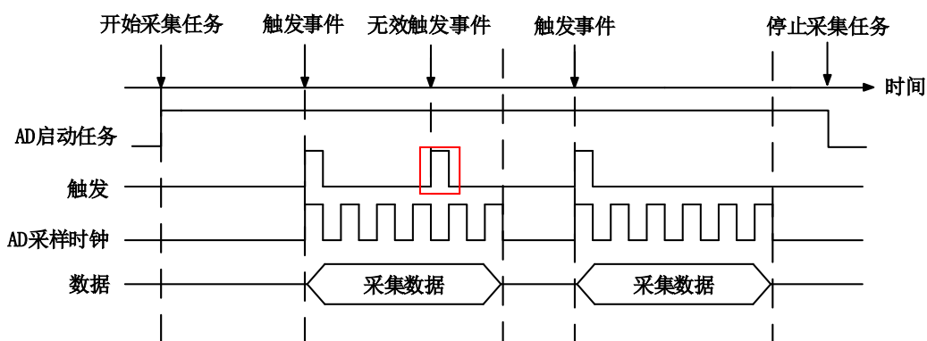
图 4-7-6 重触发
