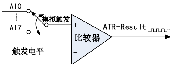
图4-8-7 比较器
