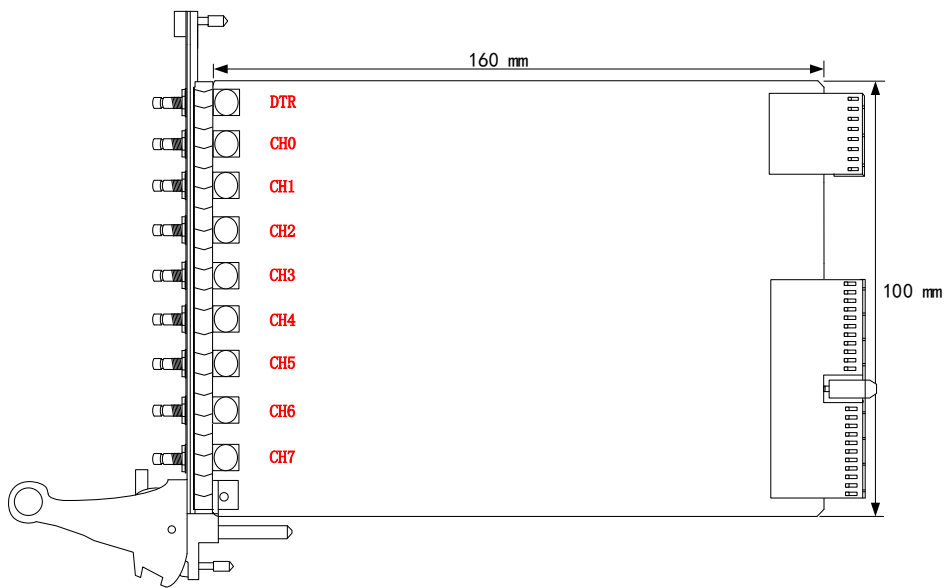
图 3-2-2 PXI8811/ PXI8814 板卡尺寸图
