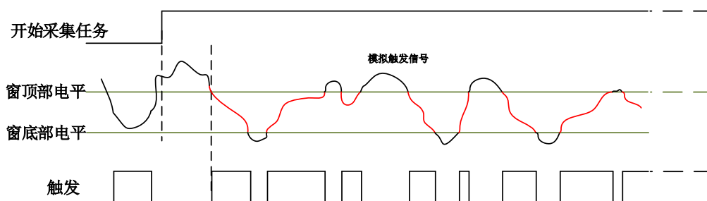
图4-8-8 模拟窗触发--入窗
