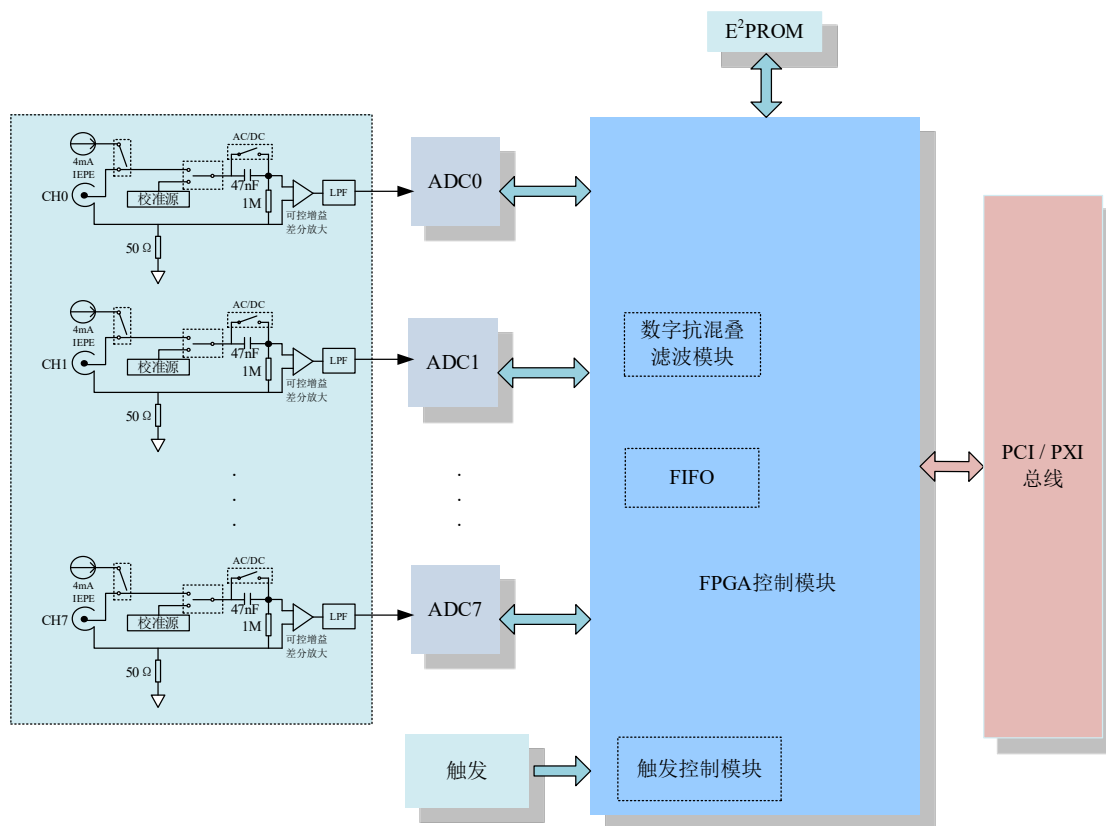
图 2-2-1 PCI/PXI 8811/8814 系统框图
