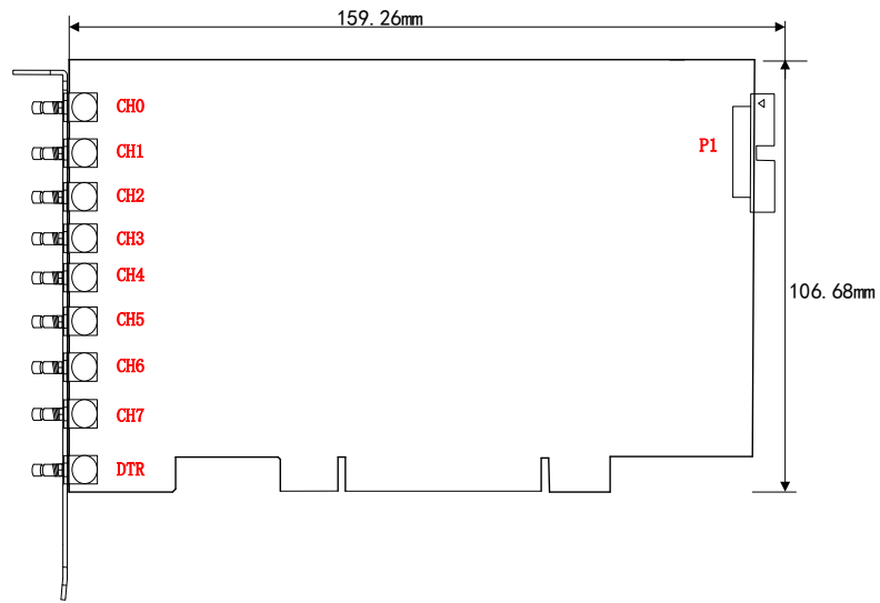
图 3-2-1 PCI8811 /PCI8814 板卡尺寸图
