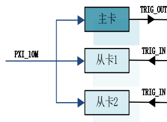
图 4-10-1 采用 PXI 机箱背板的 PXI_10M 时钟信号作为时钟参考源
