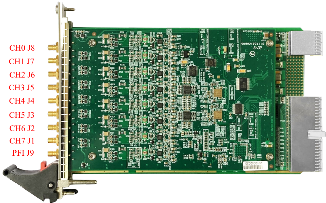
图 3-3-1 PXI8582\8584\8586 产品外观图
