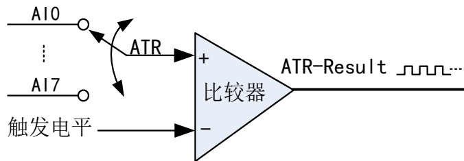
图 4-8-5 比较器
