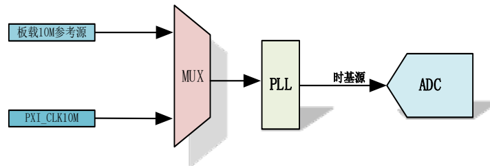
图 4-7-1 时基源框图
