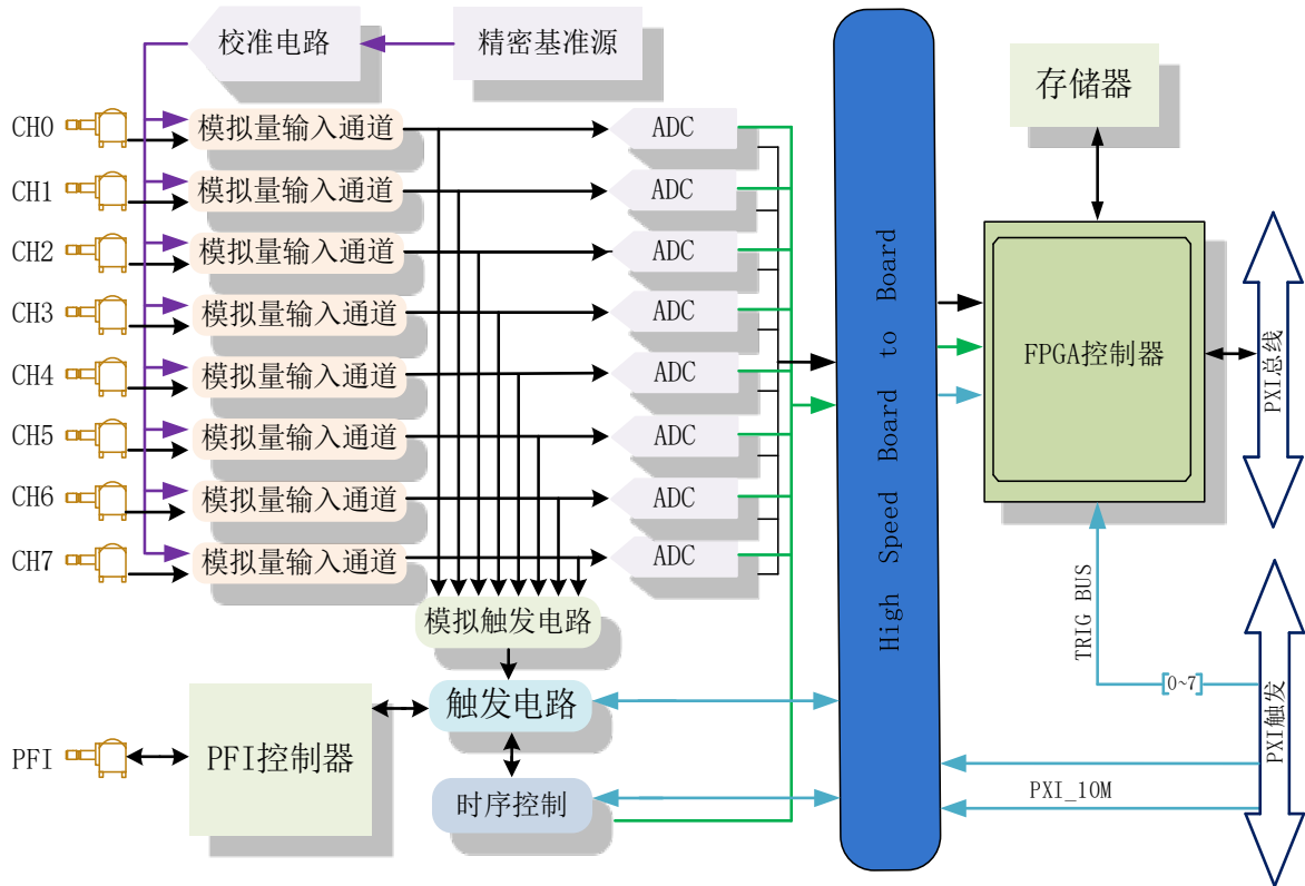
图 3-1-1 PXI8582\8584\8586 系统框图
