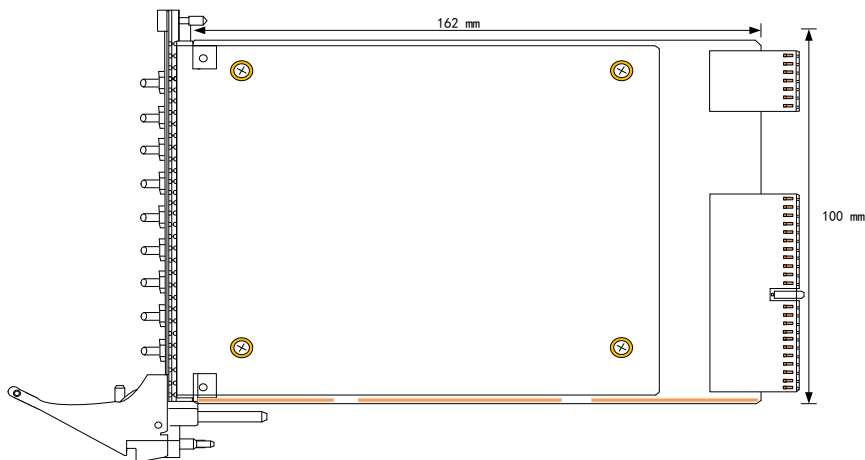
图 3-2-1 PXI8582\8584\8586 板卡尺寸图
