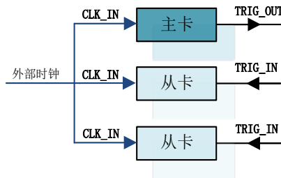
图 4-11-2 共同的外时钟
