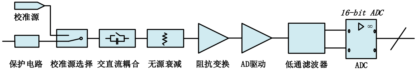
图 4-1-1 AD 功能框图
