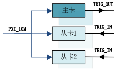
图 4-11-1 采用 PXI 机箱背板的 PXI_10M 时钟信号作为时钟参考源
