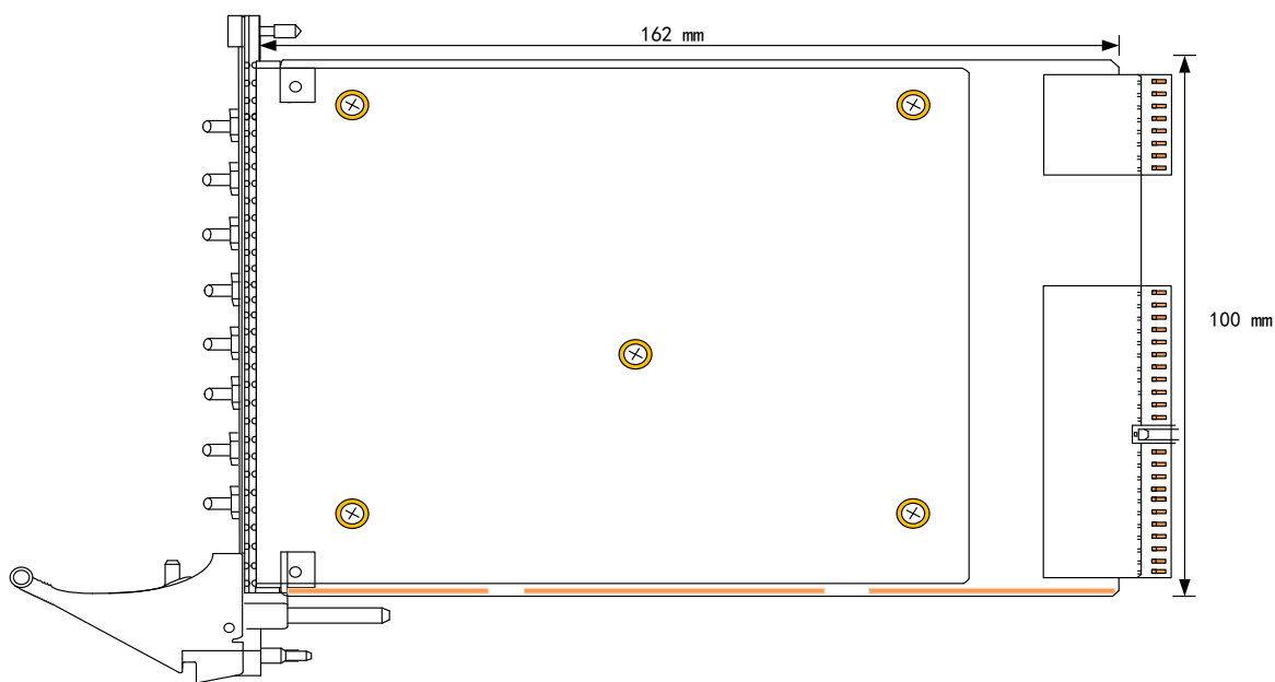
图 3-2-1 PXI8506B 板卡尺寸图
