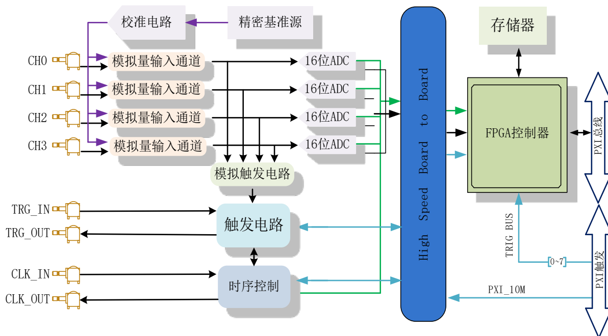
图 3-1-1 PXI8506B 系统框图
