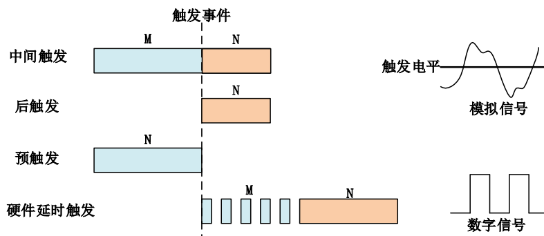
图 4-10-1 AD 触发模式
