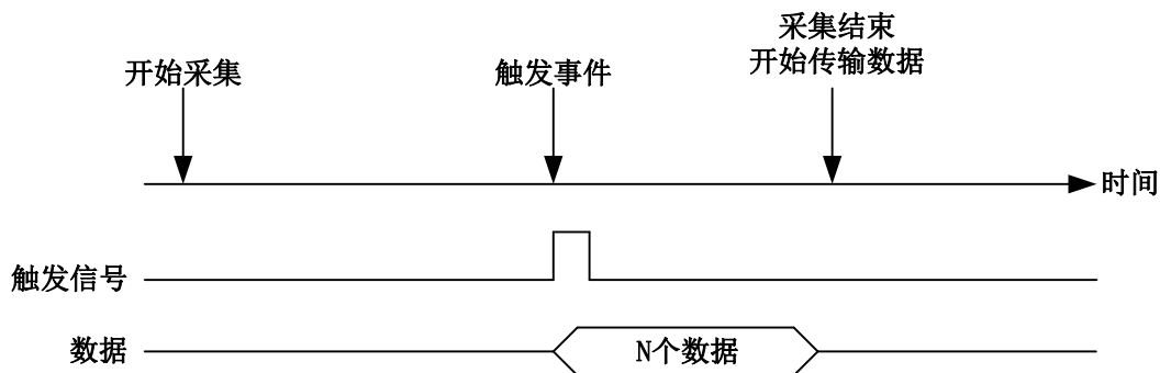
图 4-10-3 后触发
