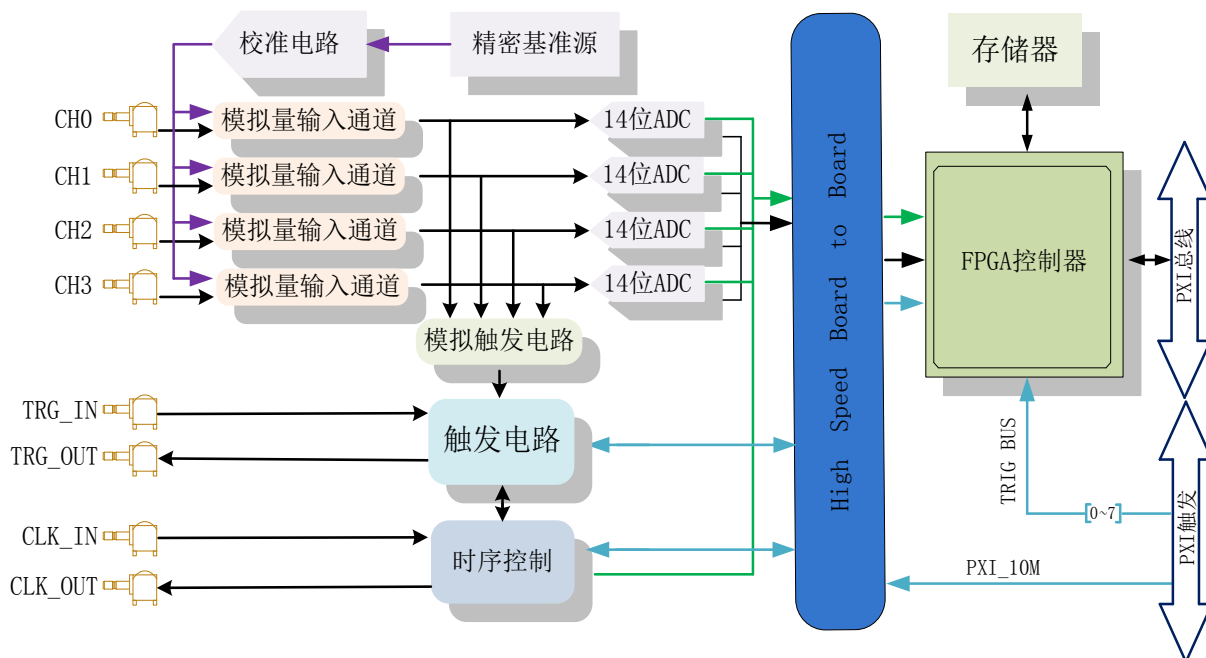
图 3-1-1 PXI8504B/8514B 系统框图
