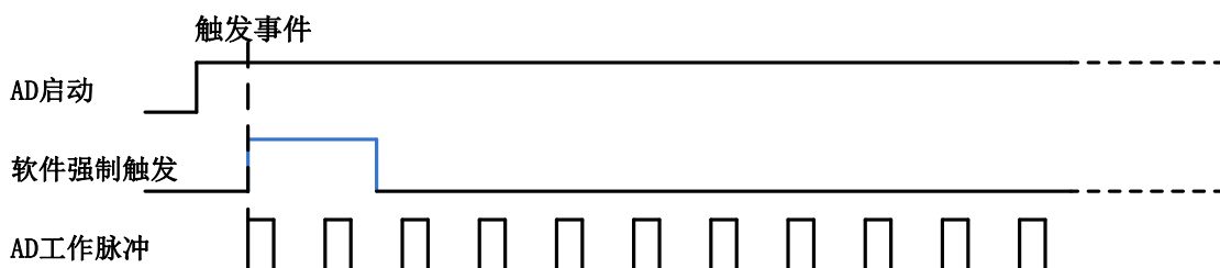
图 4-9-3 AD 软件触发
