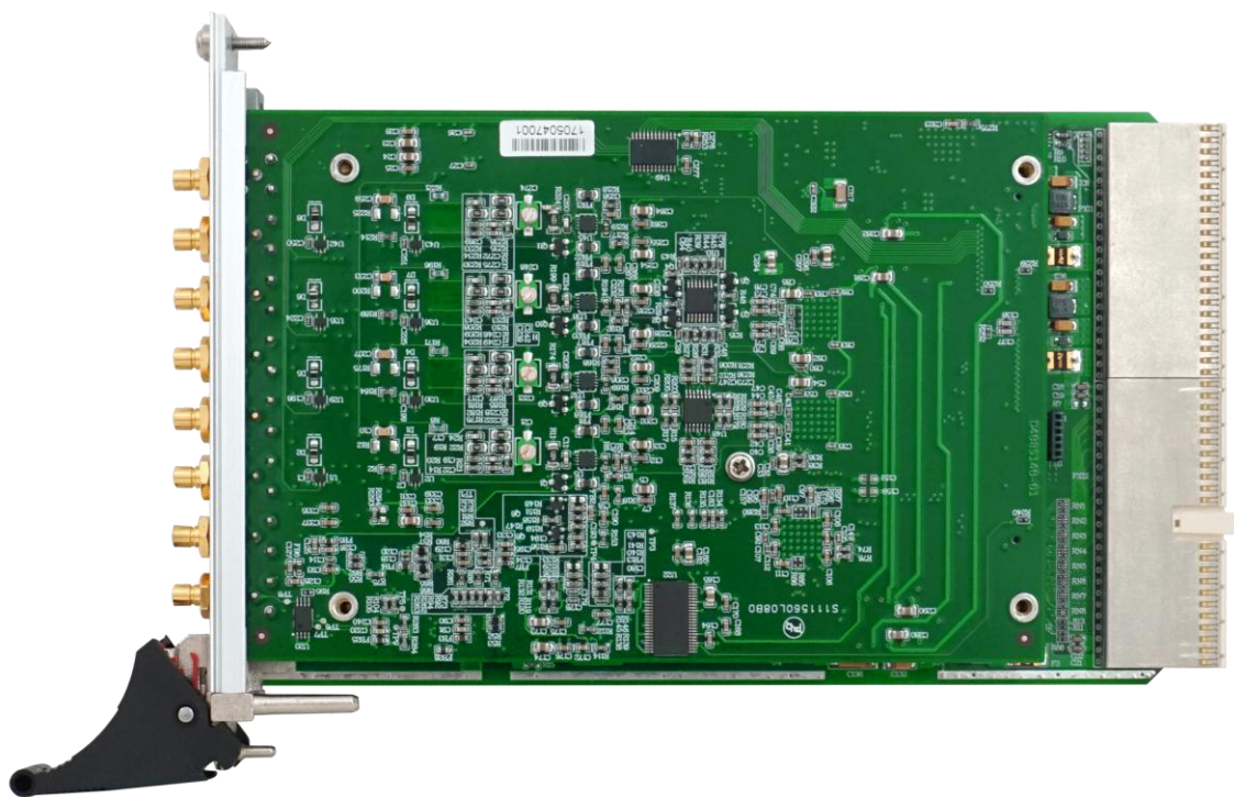
图 3-3-1 PXI8504B/8514B 元件布局图
