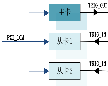
图 4-11-1 采用PXI机箱背板的PXI_10M时钟信号作为时钟参考源
