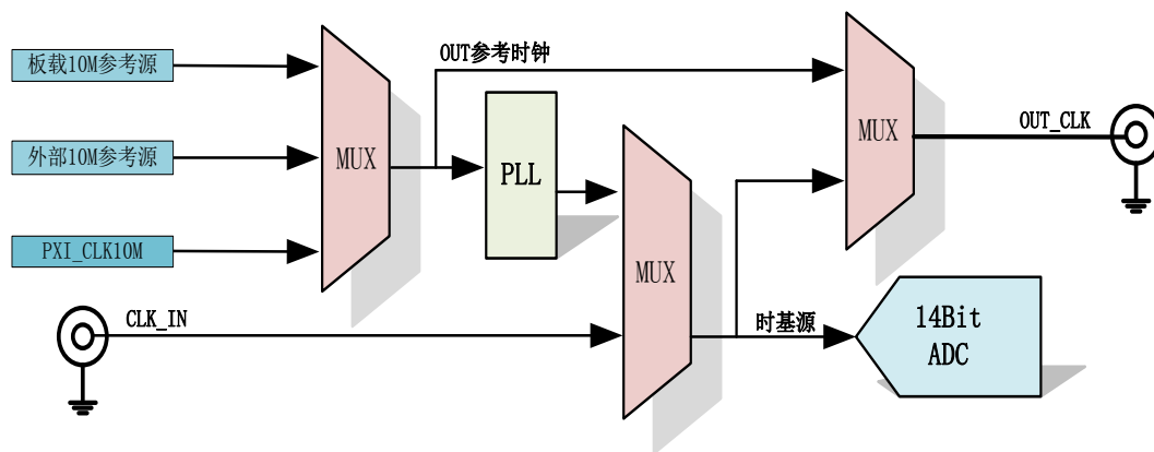
图 4-7-1 时基源框图
