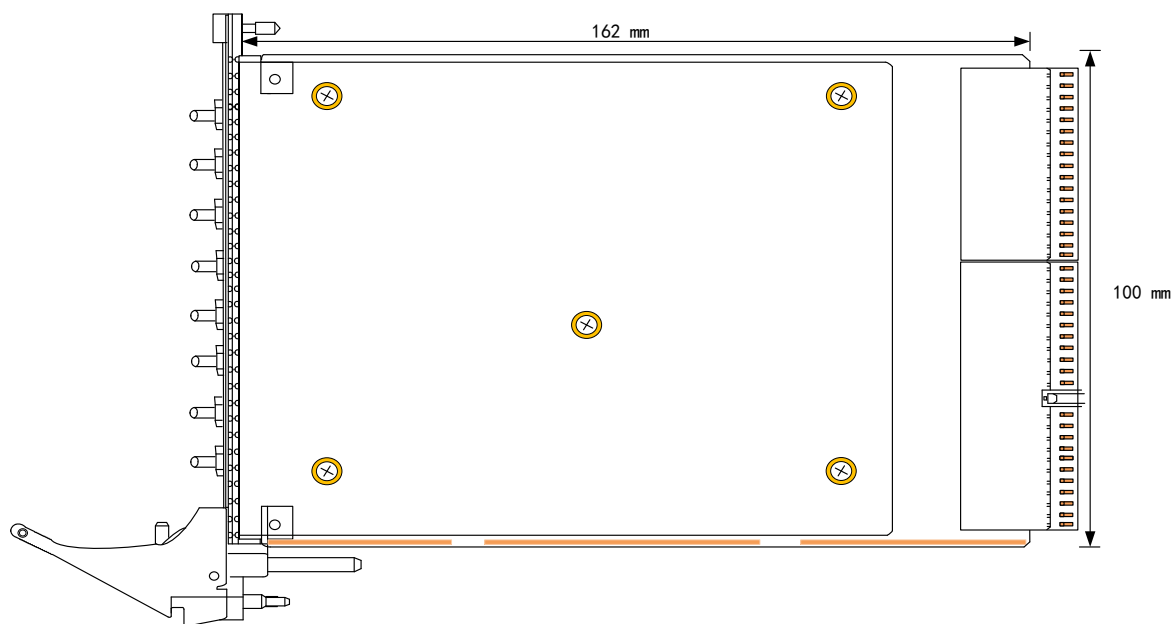
图 3-2-1 PXI-8504B/8514B 板卡尺寸图
