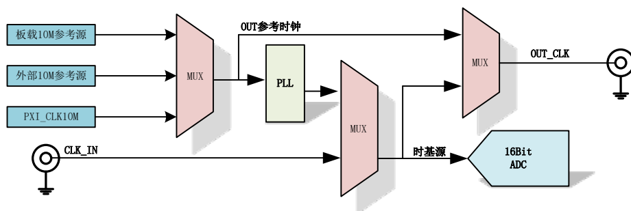
图 4-7-1 时基源框图
