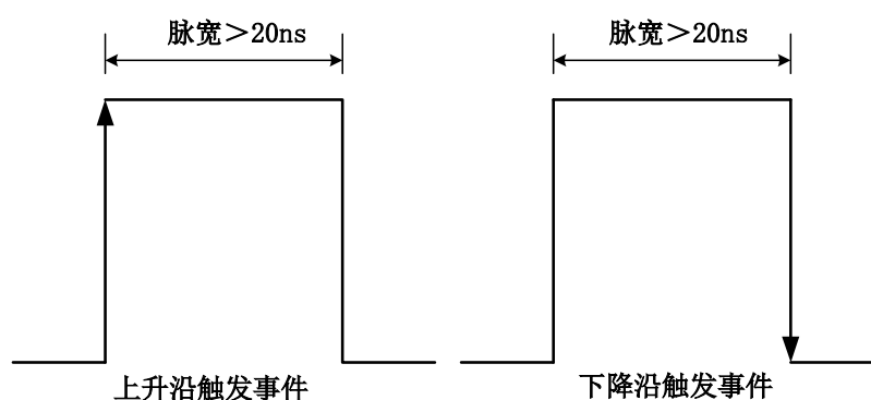
图 4-9-8 脉宽最小值图
