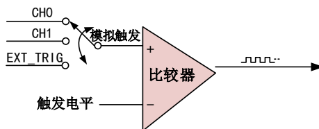
图5-3-4 比较器
