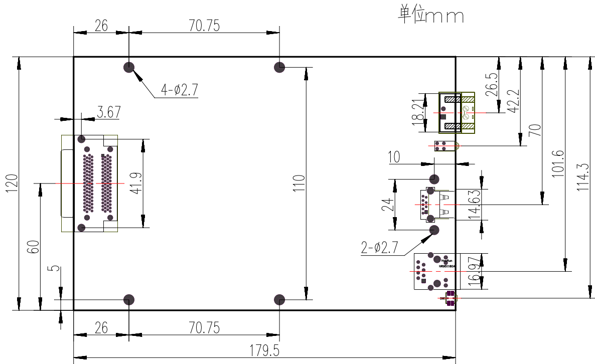
图 3-2-2 USB5633-V 内部尺寸图
