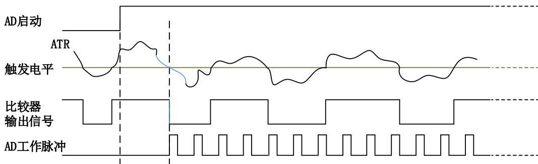
图 4-9-6 模拟触发--下降沿触发
