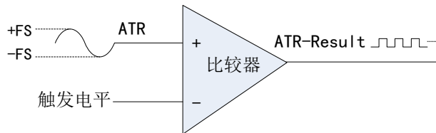
图4-9-5 比较器
