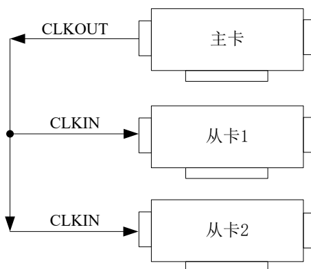
图 4-10-1 主从卡级联
