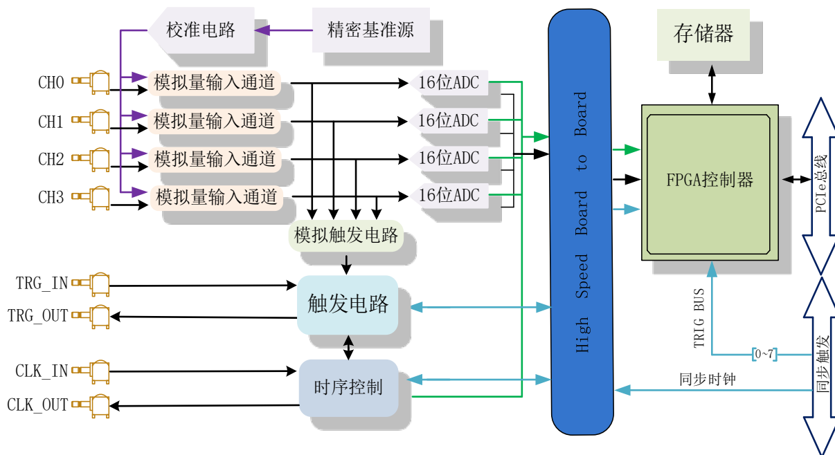
图 3-1-1 PCIe8506/8516 系统框图
