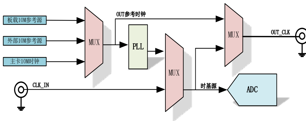
图 4-7-1 时基源框图
