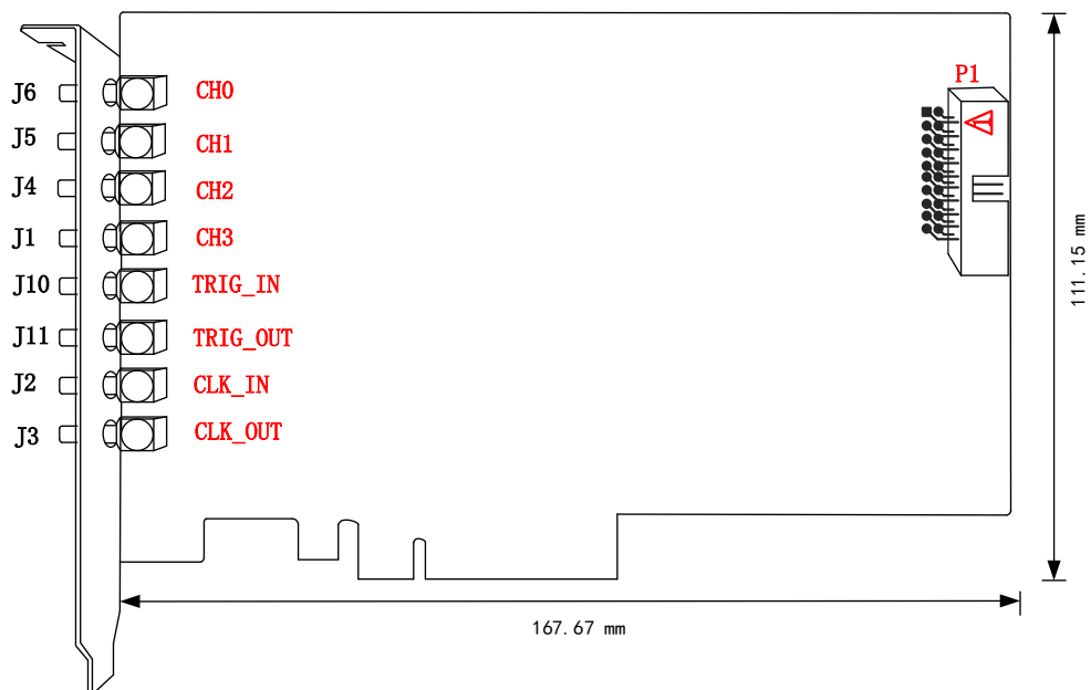
图 3-2-1 PCIe8506/8516 板卡尺寸图
