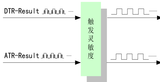
图 4-8-2 触发灵敏度
