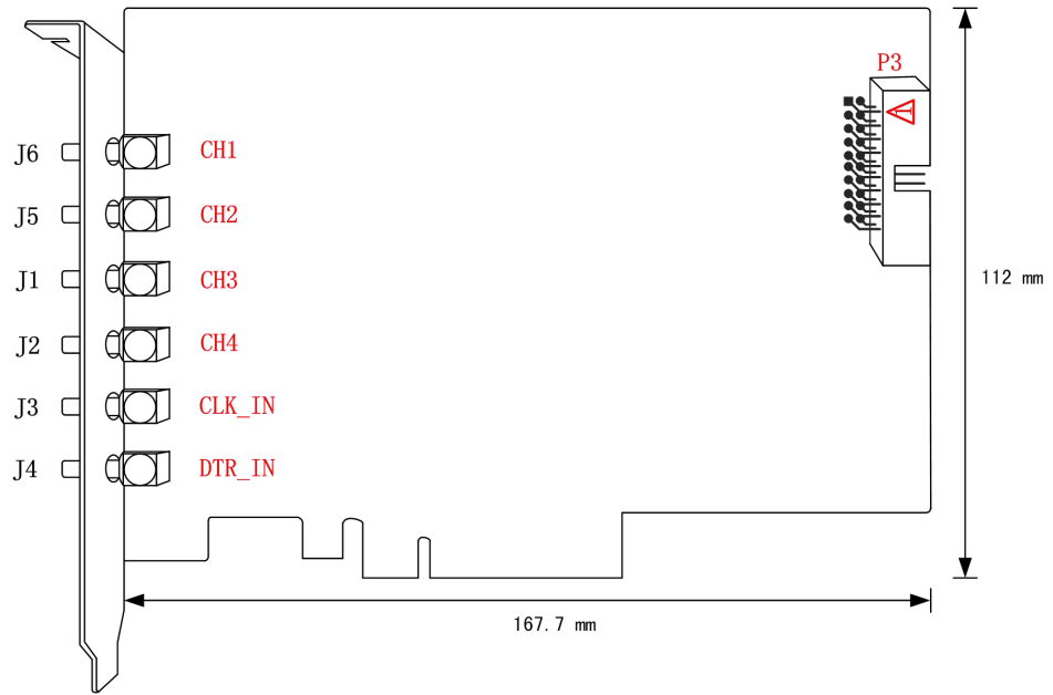
图 3-2-1 PCIe-8534B/8544B 板卡尺寸图
