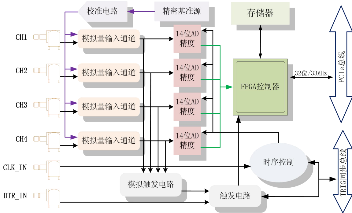
图 3-1-1 PCIe-8534B/8544B 系统框图
