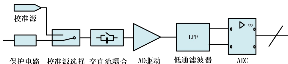
图 4-1-1 AD 功能框图
