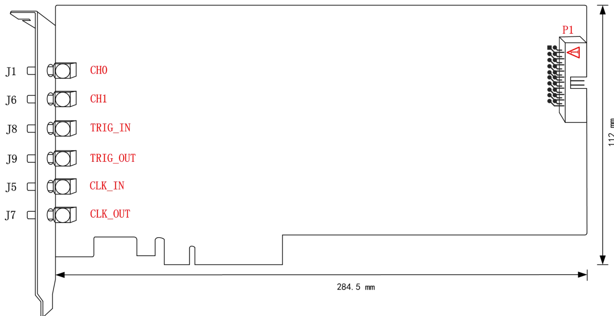
图 3-2-1 PCIe8914A\8912A 板卡尺寸图
