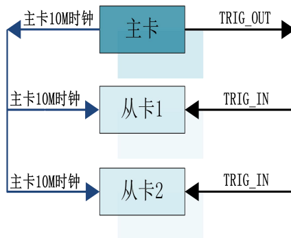
图 4-10-1 主从卡级联
