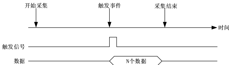
图 4-9-2-2 后触发
