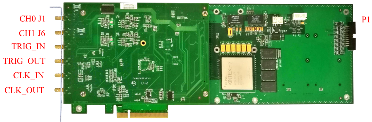
图 3-3-1 PCIe8914A\8912A 产品外观图
