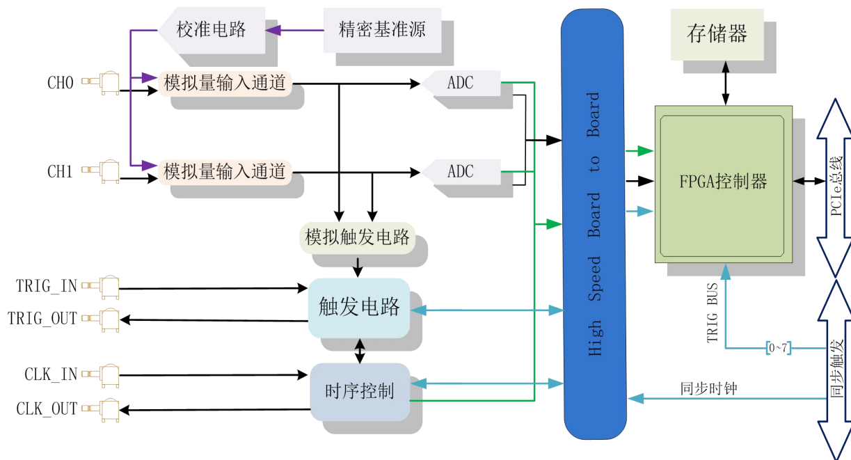
图 3-1-1 PCIe8914A\8912A 系统框图
