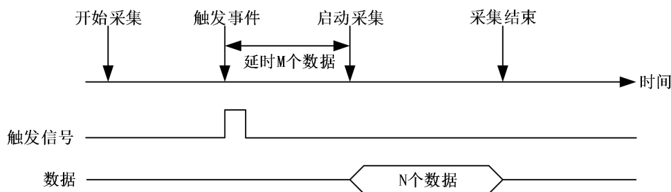
图 4-9-2-3 硬件延时触发
