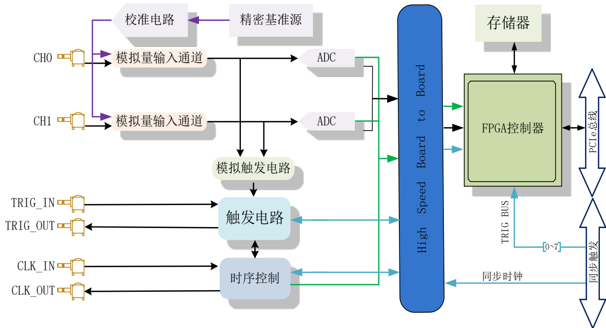
图 3-1-1 PCIe891xM 系统框图
