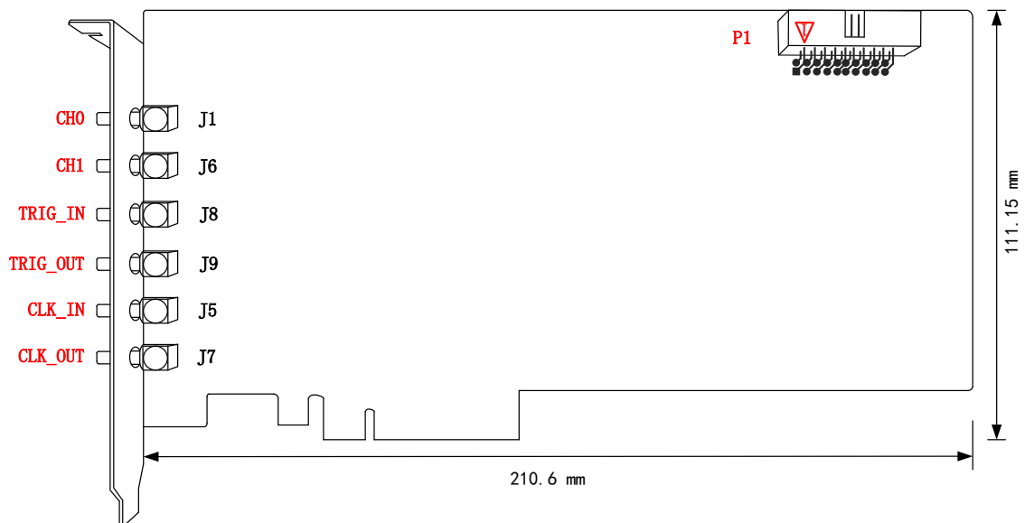
图 3-2-1 PCIe891xM 板卡尺寸图
