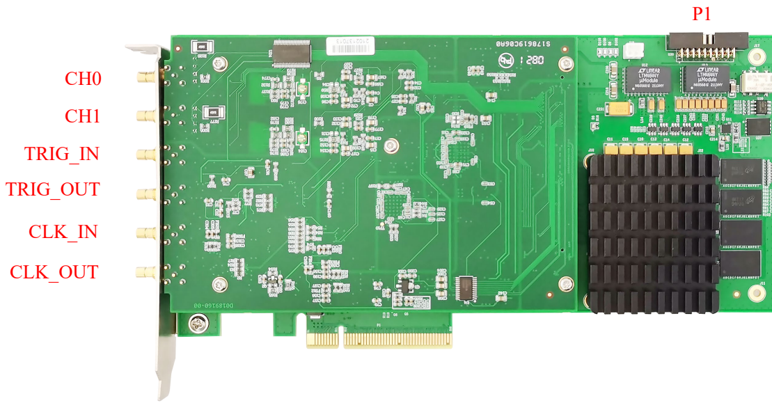
图 3-3-1 PCIe891xM 产品外观图
