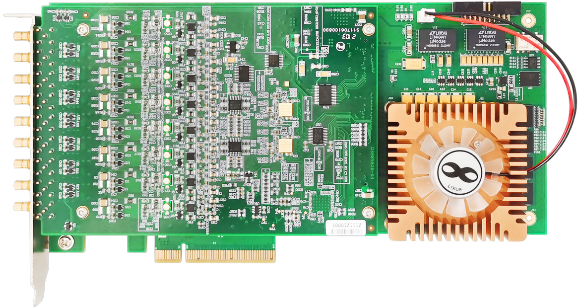
图 3-3-1 PCIe858xM 产品外观图
