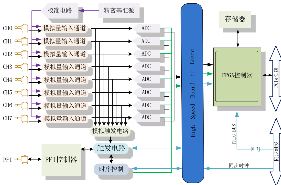
图 3-1-1 PCIe858xM 系统框图
