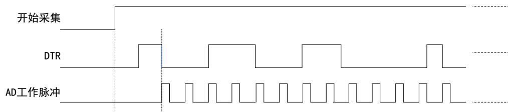
图 4-9-9 DTR 触发—下降沿触发
