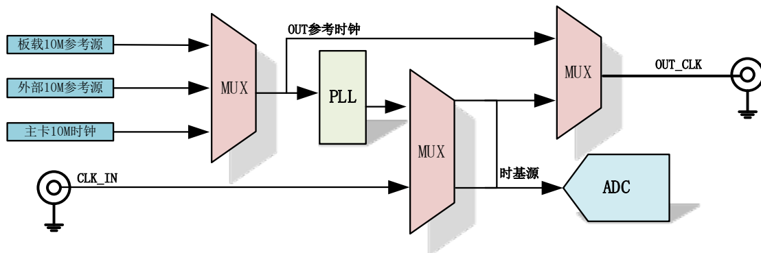
图 4-7-1 时钟选择框图
