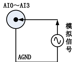
图 4-4-1 AD 信号连接
