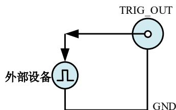
图 4-9-10 触发信号输出连接
