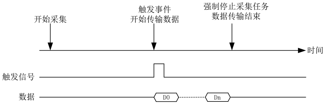
图4-8-2 后触发模式采样
