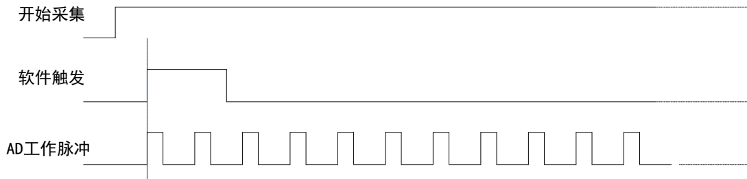
图4-9-3 AD内触发
