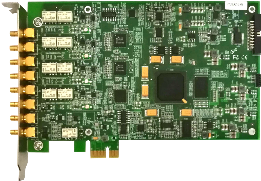
图 3-3-1 PCIe8532BL 产品外观图
