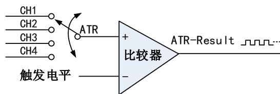
图4-9-5 比较器
