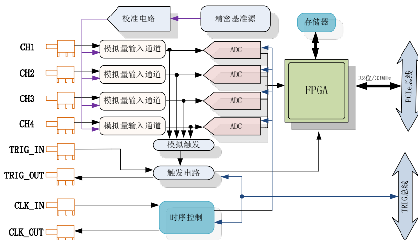
图 3-1-1 PCIe8532BL 系统框图
