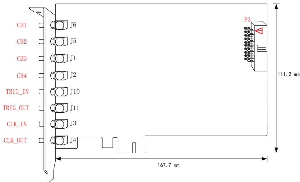
图 3-2-1 PCIe8532BL 板卡尺寸图
