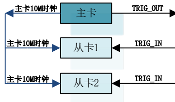
图 4-10-1 主从卡级联
