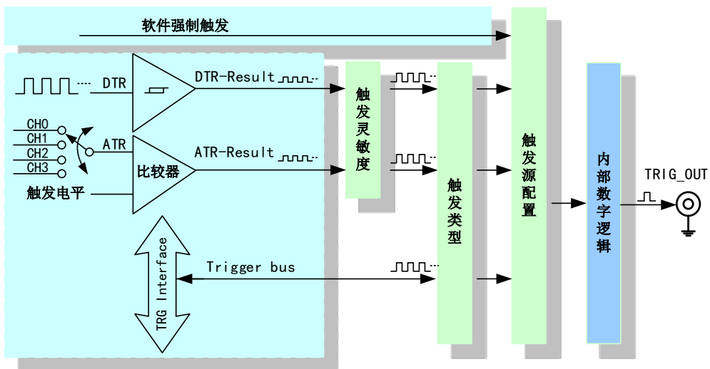
图 4-9-1 AD 触发功能框图
