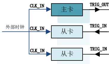
图 4-10-2 采用共同外时钟
