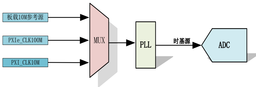
图 4-7-1 时基源框图
