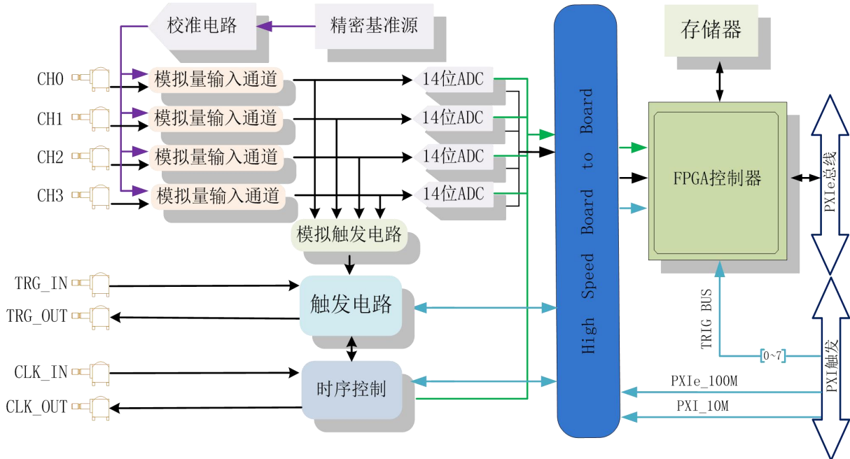
图 3-1-1 PXIe8504\8514 系统框图
