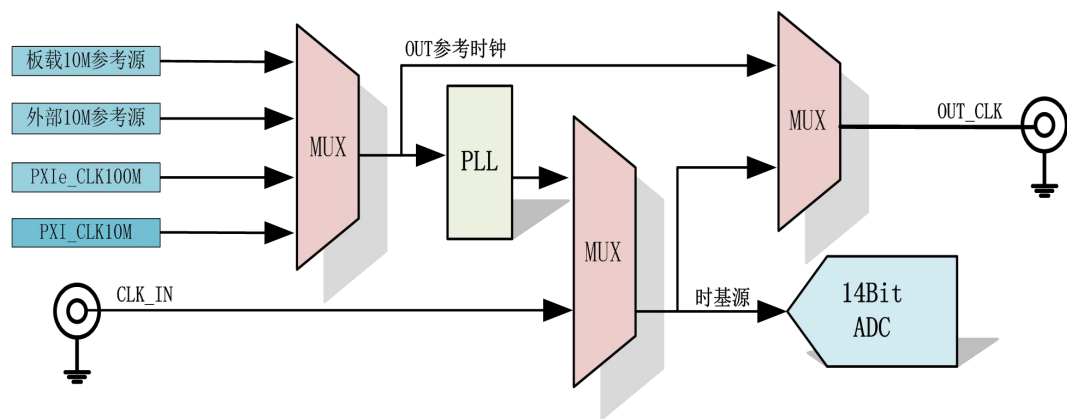
图 4-7-1 时基源框图
