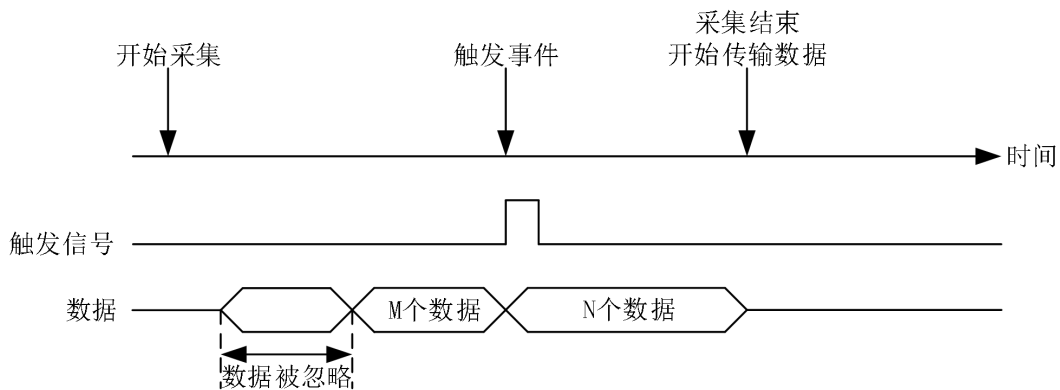
图 4-9-2-2 中间触发
