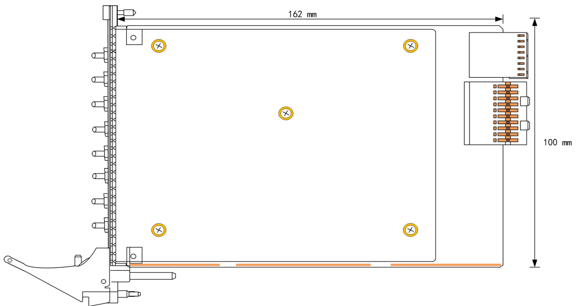
图 3-2-1 PXIe8504\8514 板卡尺寸图
