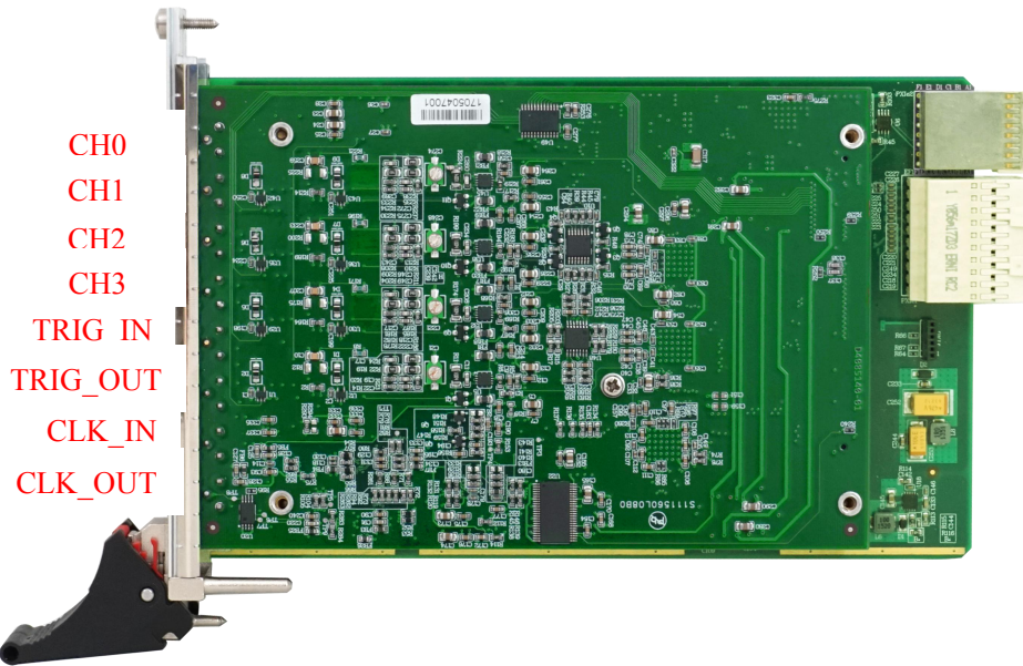
图 3-3-1 PXIe8504/8514 产品外观图
