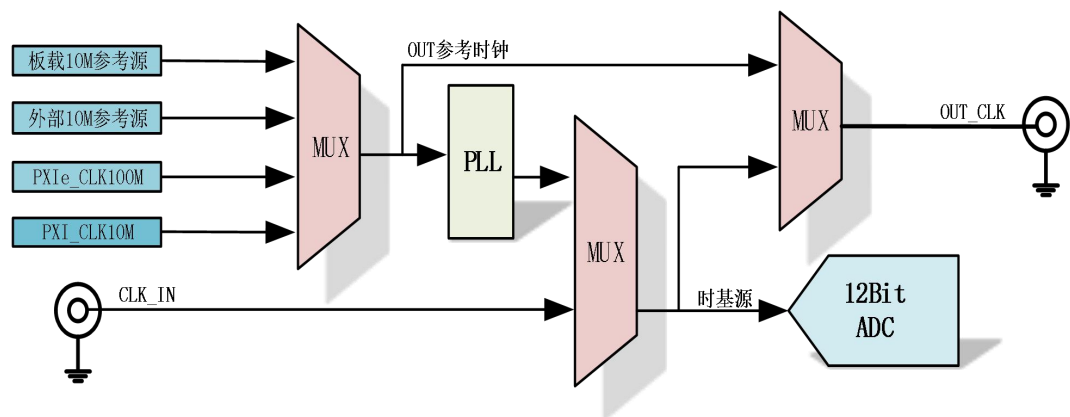
图 4-7-1 时基源框图
