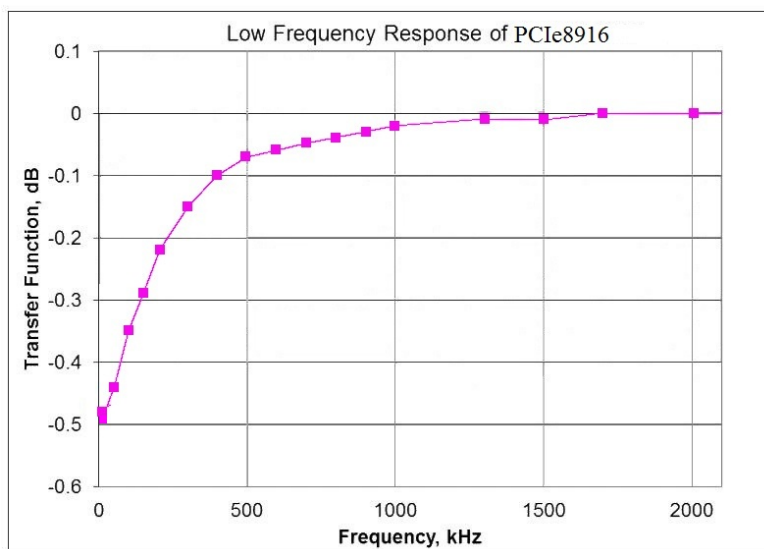
图 4-1-2 PXIe8916 低频响应
