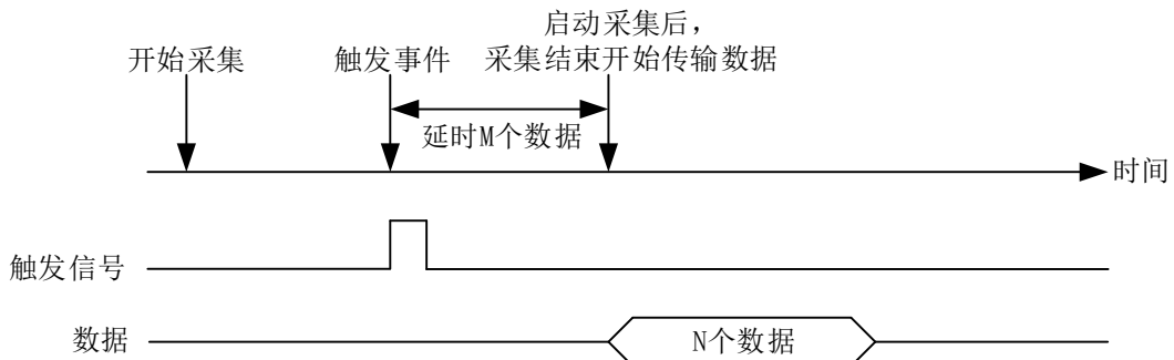
图 4-9-2-6 硬件延时触发
