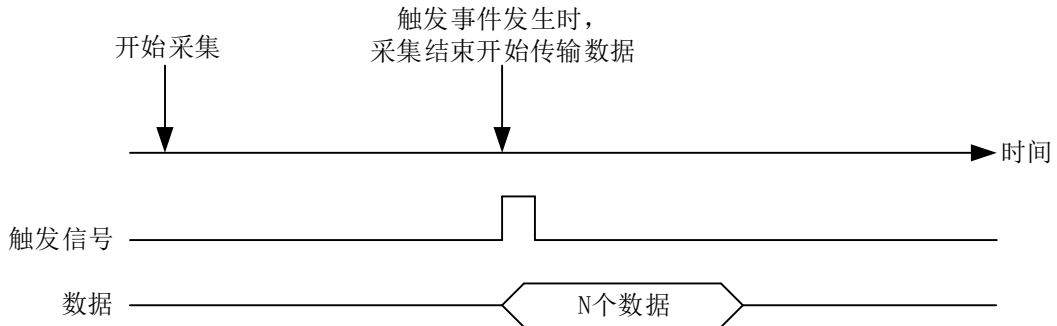
图 4-9-2-3 后触发
