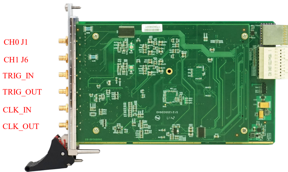
图 3-3-1 PXIe8916 产品外观图
