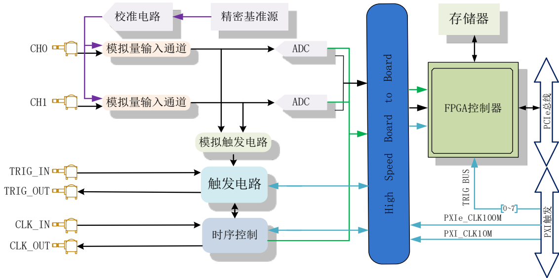
图 3-1-1 PXIe8916 系统框图
