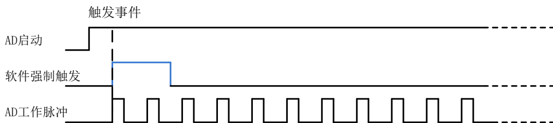
图 4-8-3 AD 软件触发
