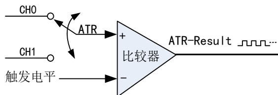
图 4-8-5 比较器
