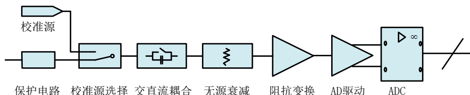
图 4-1-1 AD 功能框图
