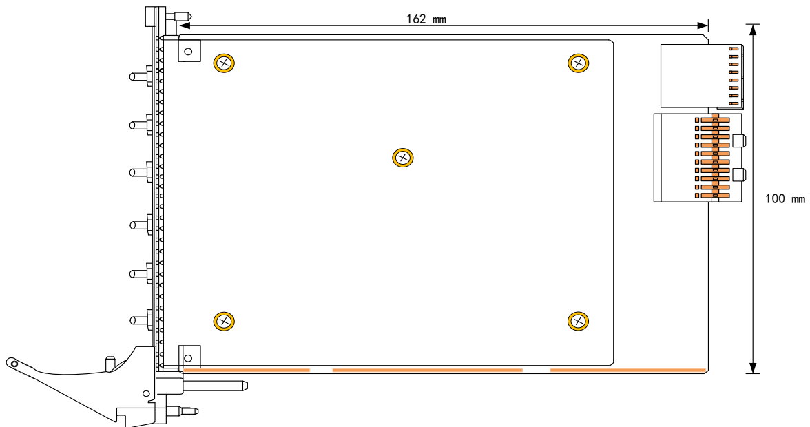
图 3-2-1 PXIe8916 板卡尺寸图
