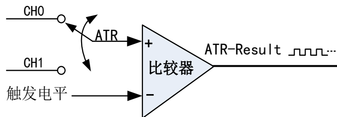
图 4-9-5 比较器
