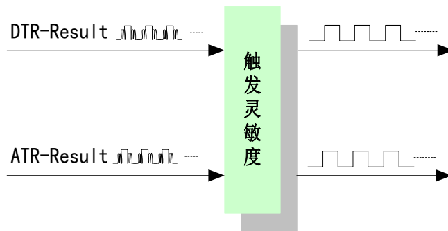
图 4-9-2 触发灵敏度
