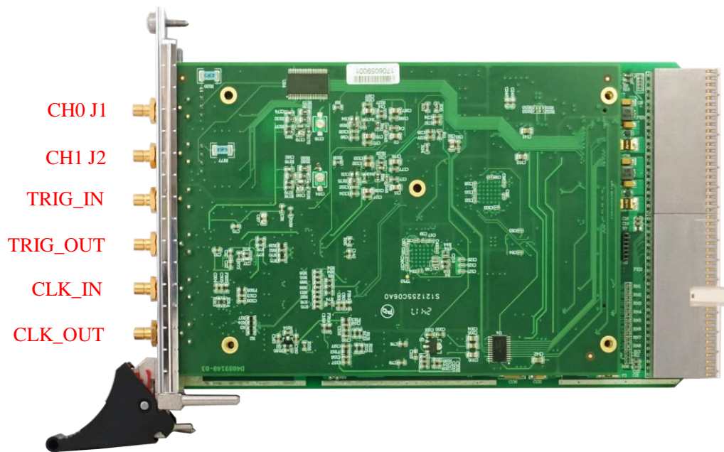
图 3-3-1 PXI8914/8912 产品外观图
