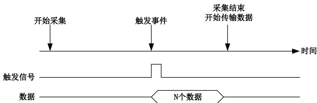
图 4-10-3 后触发
