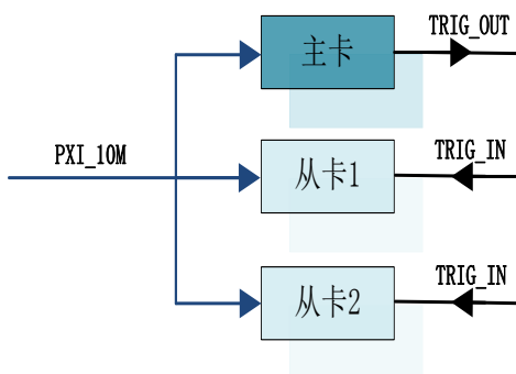
图 4-11-1 采用 PXI 机箱背板的 PXI_10M 时钟信号作为时钟参考源
