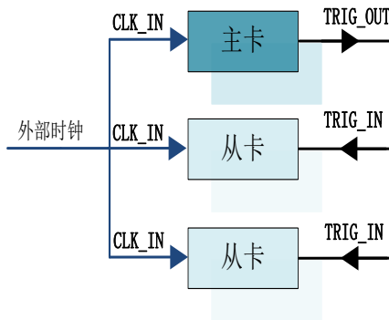
图 4-11-2 共同的外时钟
