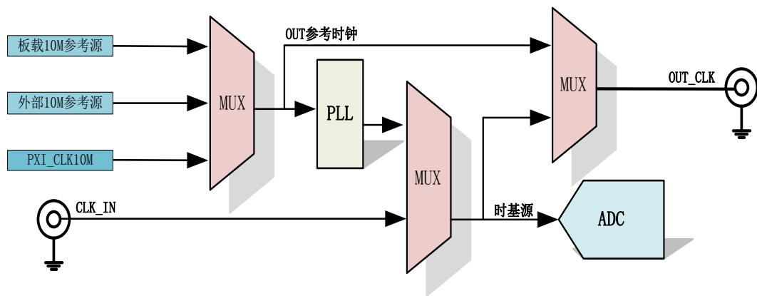
图 4-7-1 时基源框图
