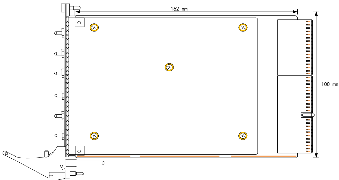
图 3-2-1 PXI8914/8912 板卡尺寸图
