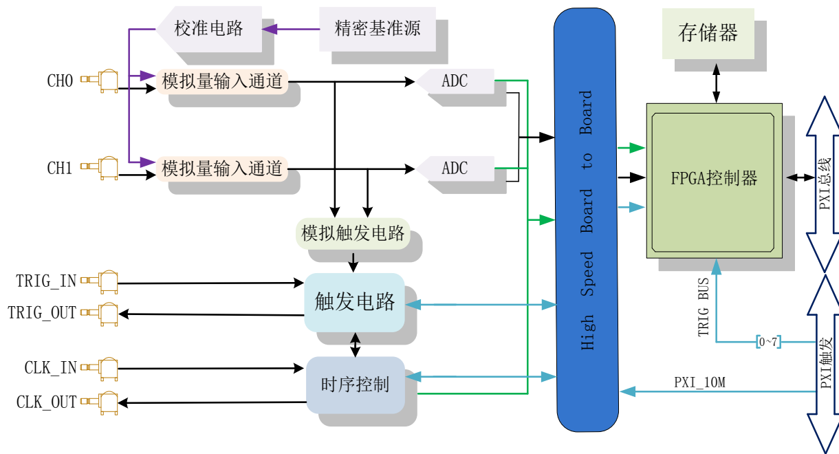
图 3-1-1 PXI8914/8912 系统框图
