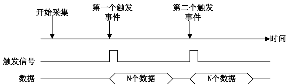
图 4-10-7 后触发和延时触发的重复触发
