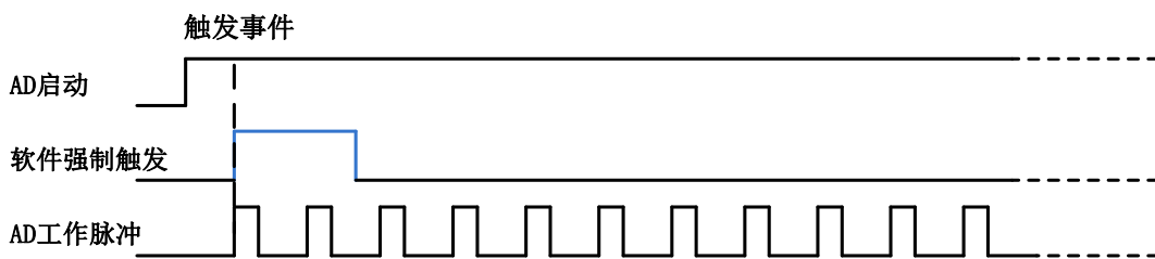
图 4-9-3 AD 软件触发
