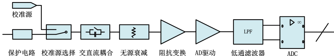
图 4-1-1 AD 功能框图
