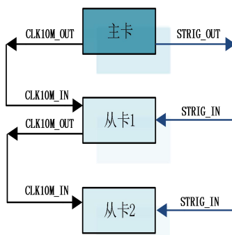
图 4-10-1 主从卡级联
