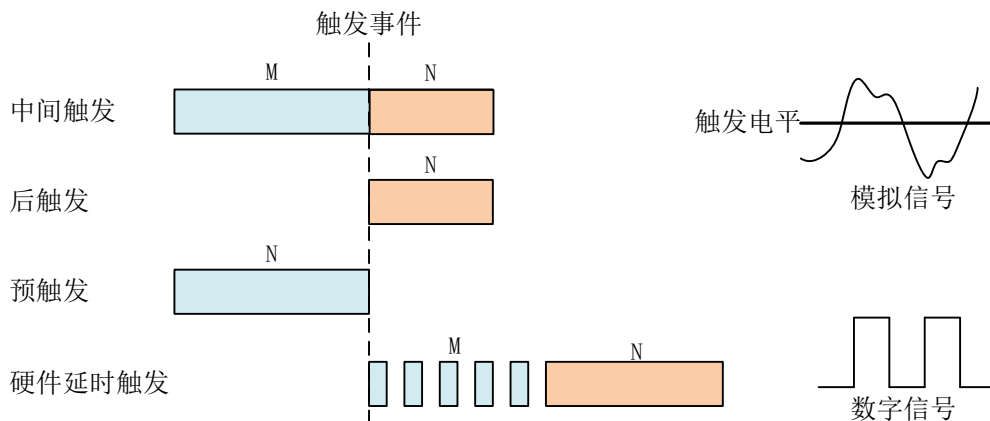
图 4-8-1-1 AD 触发模式
