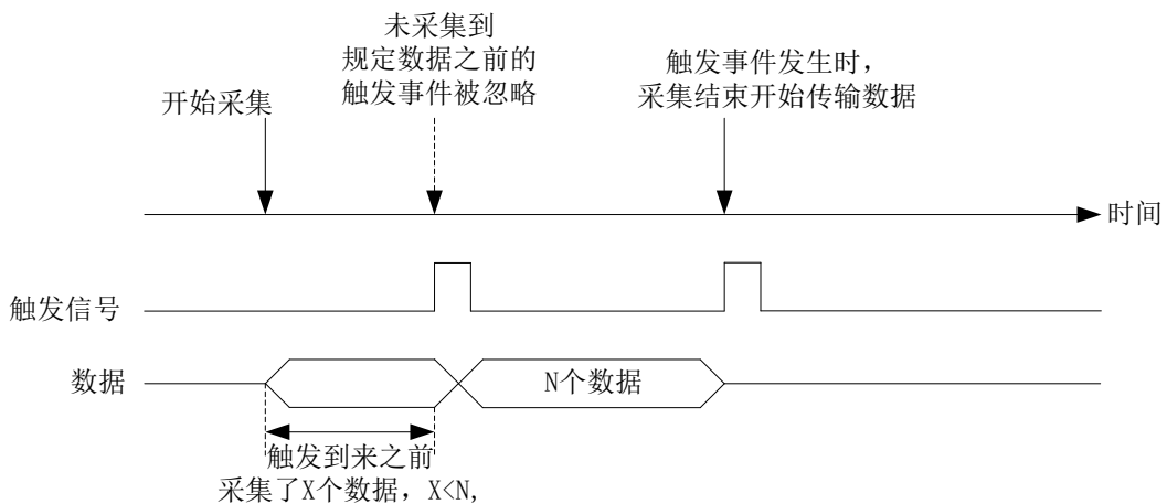
图 4-8-1-5 预触发--采集数据小于 N
