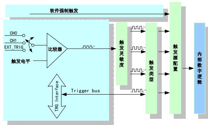
图 5-1-1 AD 触发功能框图
