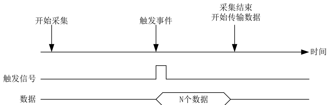
图 4-8-1-3 后触发
