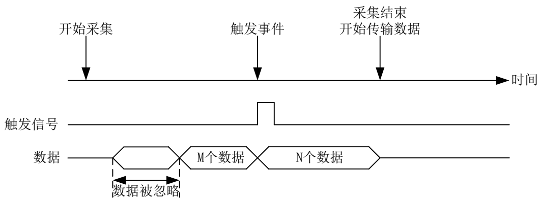
图 4-8-1-2 中间触发
