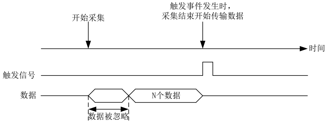
图 4-8-1-4 预触发
