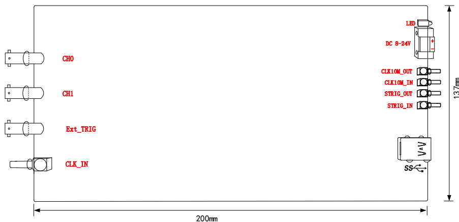
图 3-2-1 USB8910 板卡尺寸图
