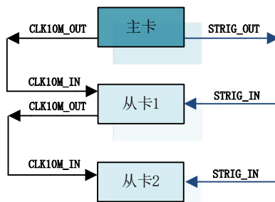
图4-10-1 主从卡级联
