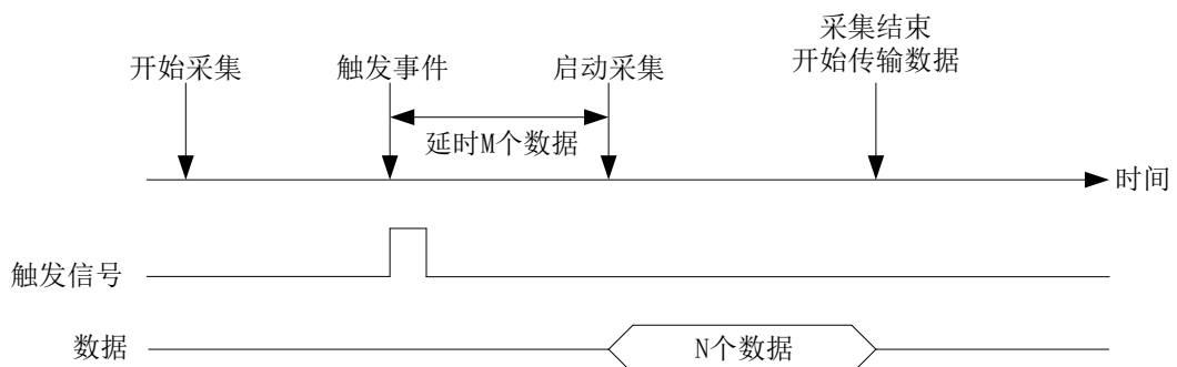
图 4-8-1-6 硬件延时触发
