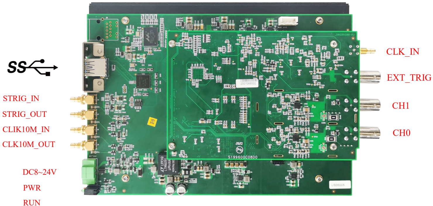
图 3-3-1 USB8910 产品外观图
