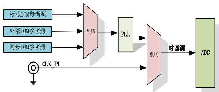
图 4-7-1 时基源框图
