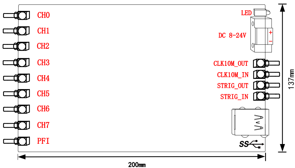
图 3-2-1 USB8582\8584\8586 板卡尺寸图
