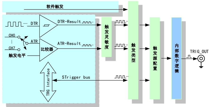
图 4-8-1 AD 触发功能框图
