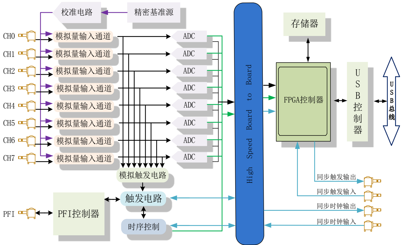
图 3-1-1 USB8582\8584\8586 系统框图
