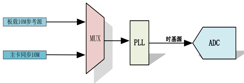
图 4-7-1 时基源框图
