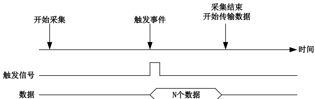
图 4-9-2-3 后触发
