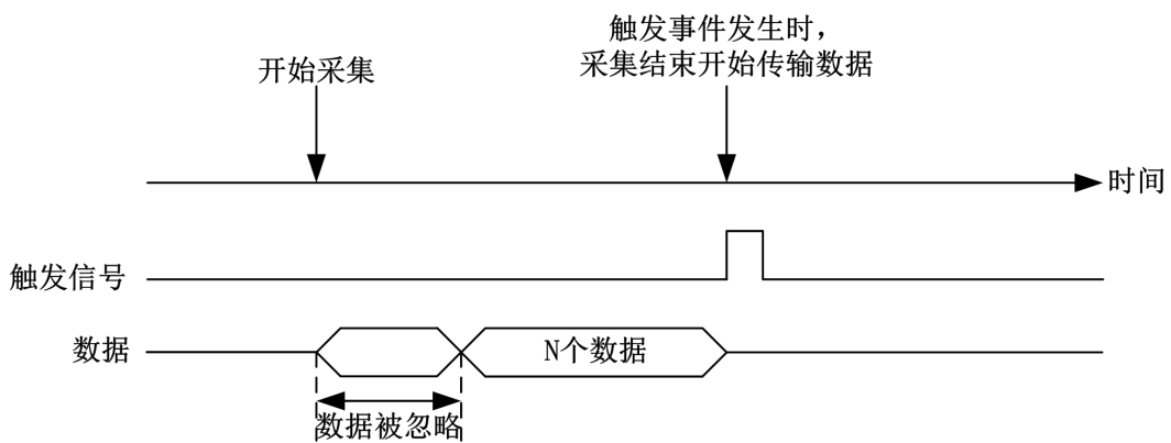
图 4-9-2-4 预触发
