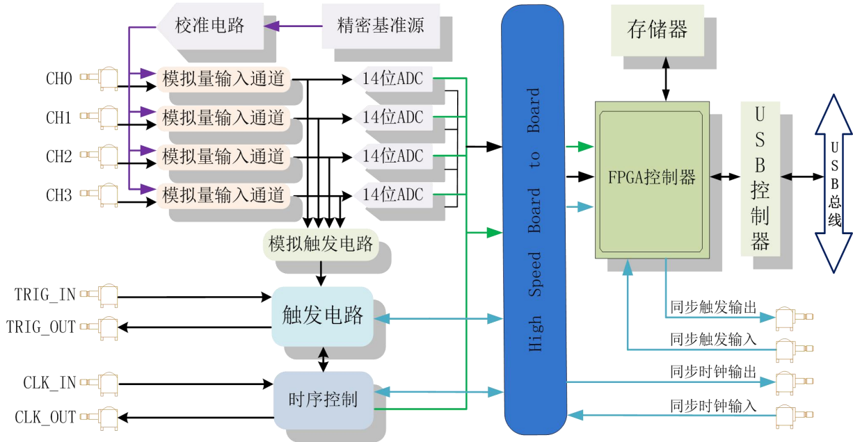
图 3-1-1 USB8504\8514 系统框图
