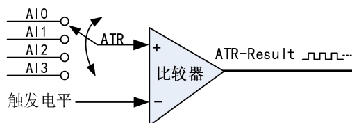
图 4-8-5 比较器
