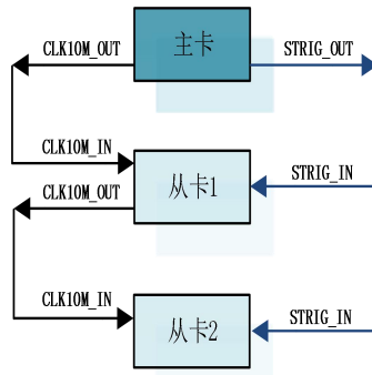
图 4-10-1 主从卡级联
