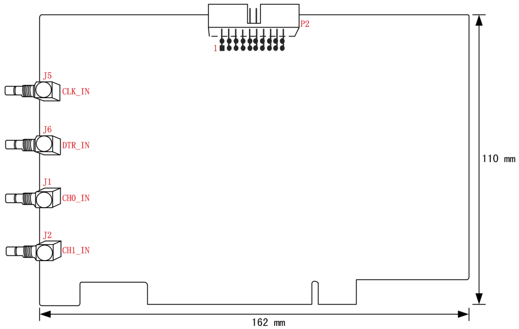
图 3-1-1 PCI8552B 板卡尺寸图
