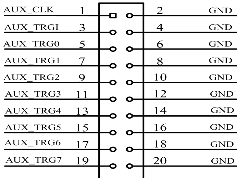
图 3-3-1 P2 管脚定义
