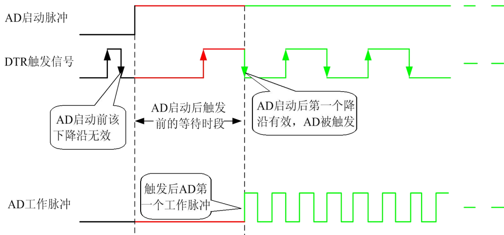
6.4 下降沿触发图例
