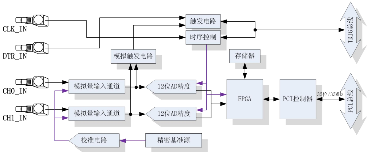
图 2-2-1 PCI8552B 系统框图
