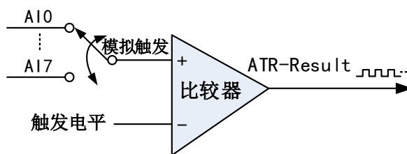
图4-8-7 比较器
