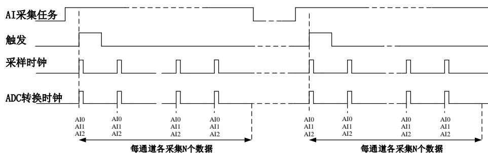
图4-6-2 有限点采样
