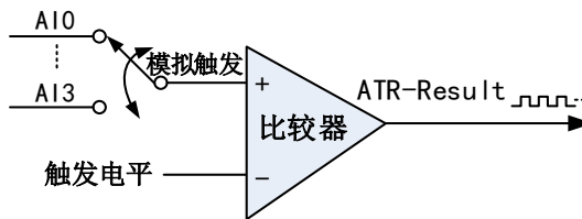
图4-8-7 比较器
