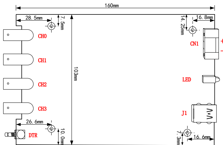
图 3-2-1 板卡尺寸图
