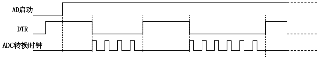
图 4-7-6 暂停触发—高电平暂停
