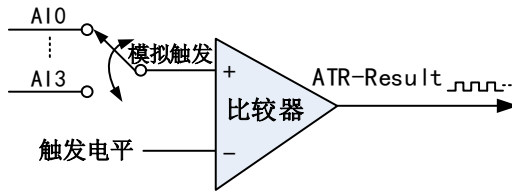
图4-8-5 比较器
