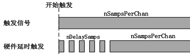
图 4-7-1 AI 触发模式
