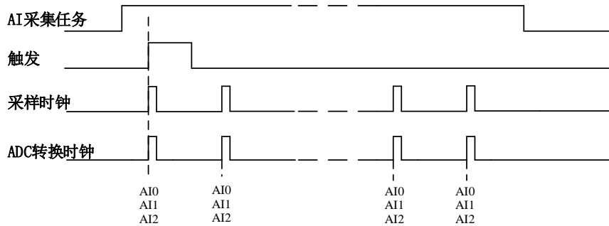
图4-6-3 连续采样
