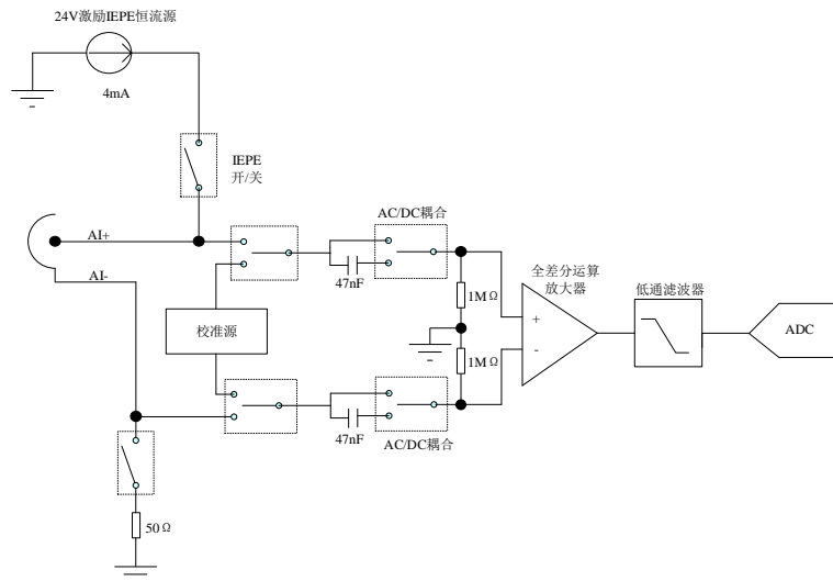
图 4.1.1 模拟输入功能框图
