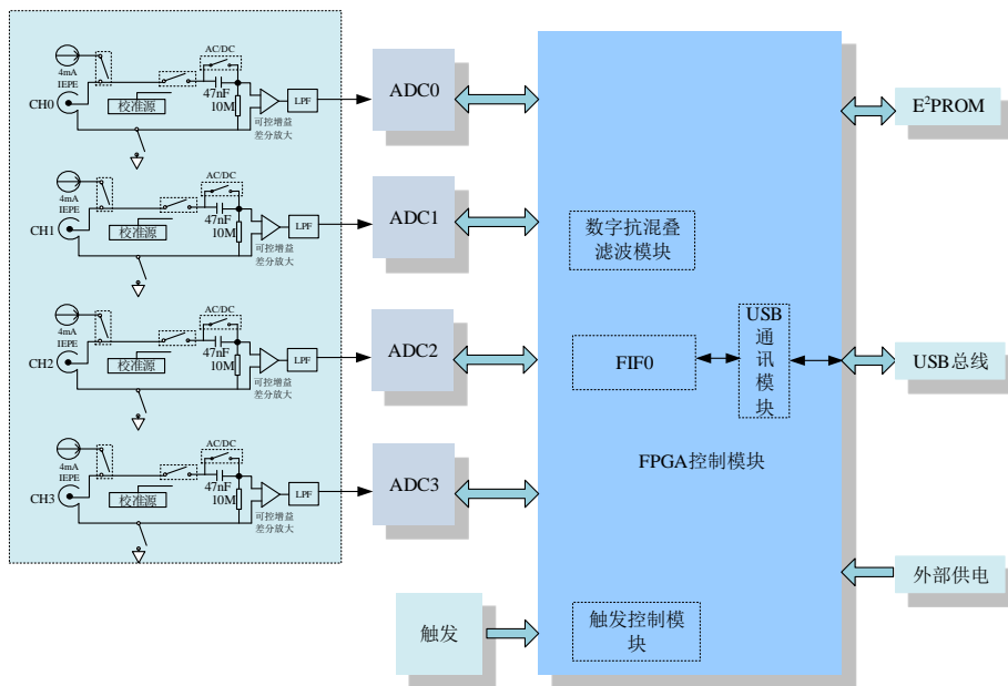
图 2.2.1 USB8812 系统框图
