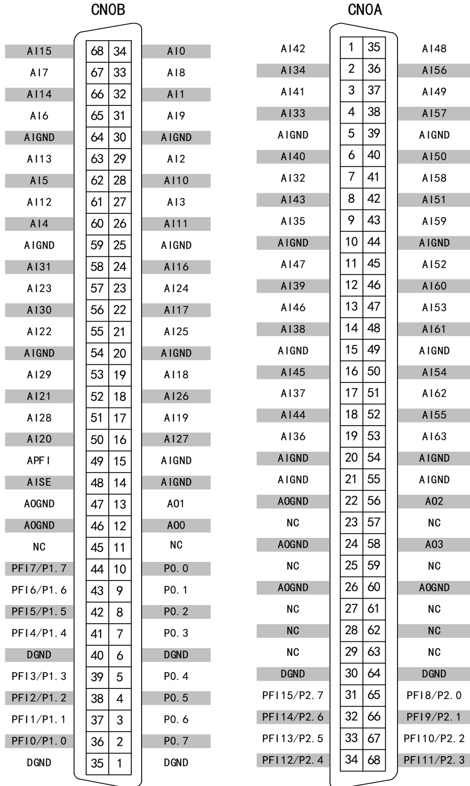
图 3-3-1 连接器引脚定义
