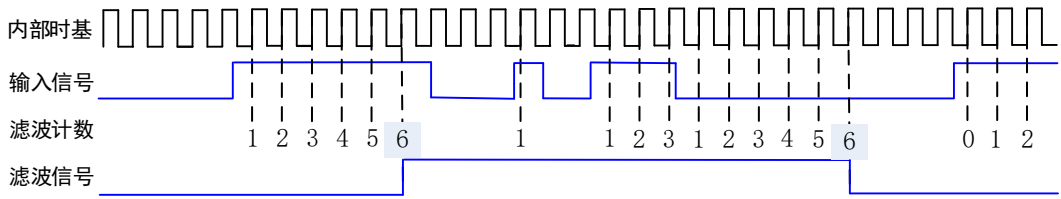
图 6-9-1 数字滤波
