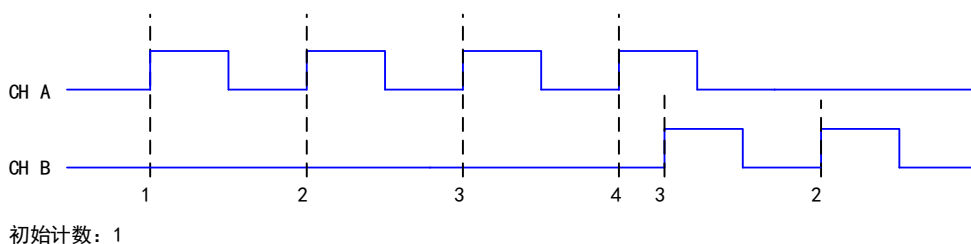
图 6-7-4 双脉冲编码
