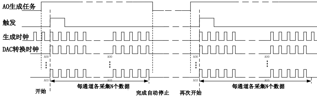
图5-7-2 内、外时钟有限点生成
