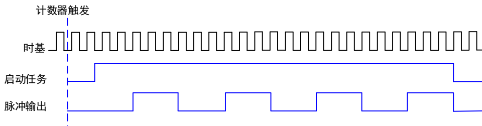
图 6-8-3 有限脉冲序列生成
