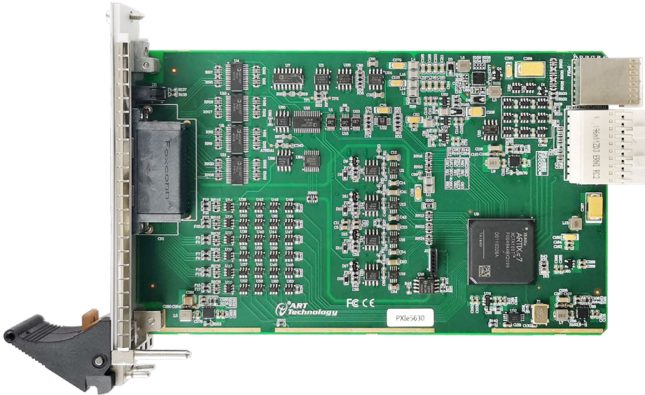
图 3-1-1 PXIe5630 正面图
