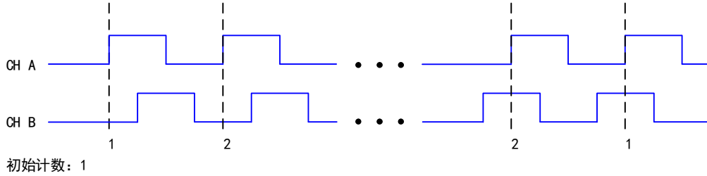
图 6-7-1 X1 编码
