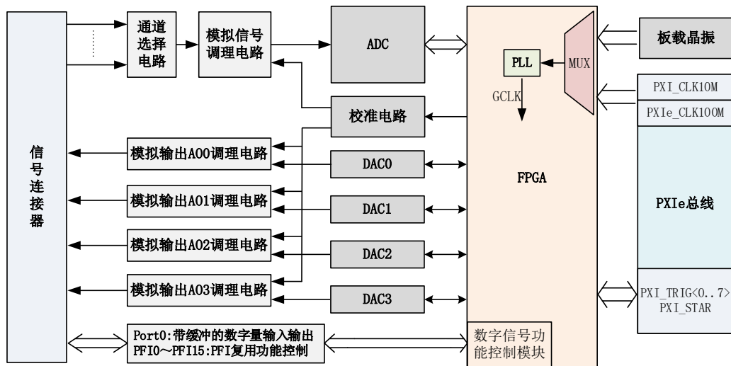
图2-2-1 PXIe5630系统框图
