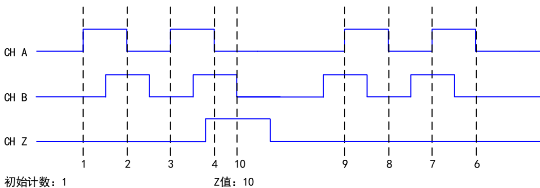
图 6-7-6 Z 索引
