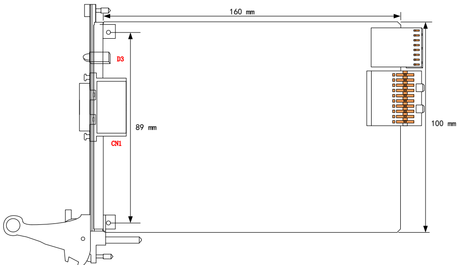
图 3-2-1 外壳尺寸图
