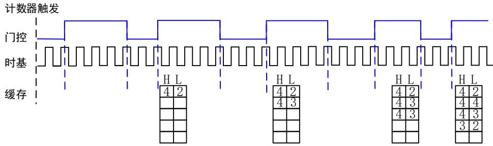
图 6-4-2 隐式缓冲脉冲测量
