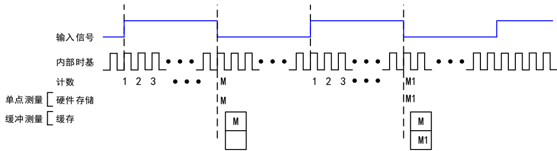
图 6-5-1 脉宽测量上升沿有效示意图
