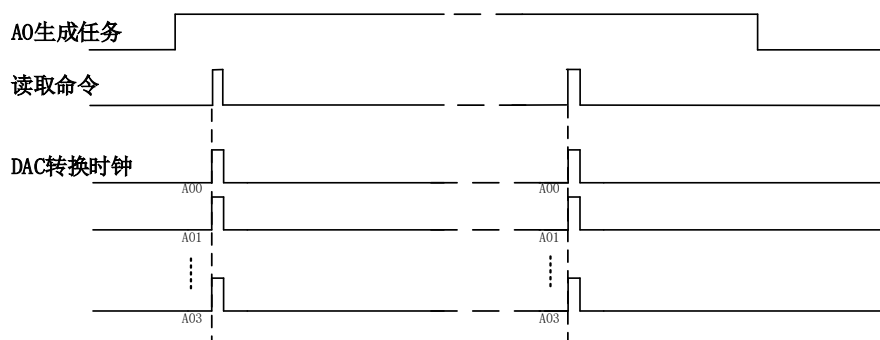
图5-7-1 按需单点采集
