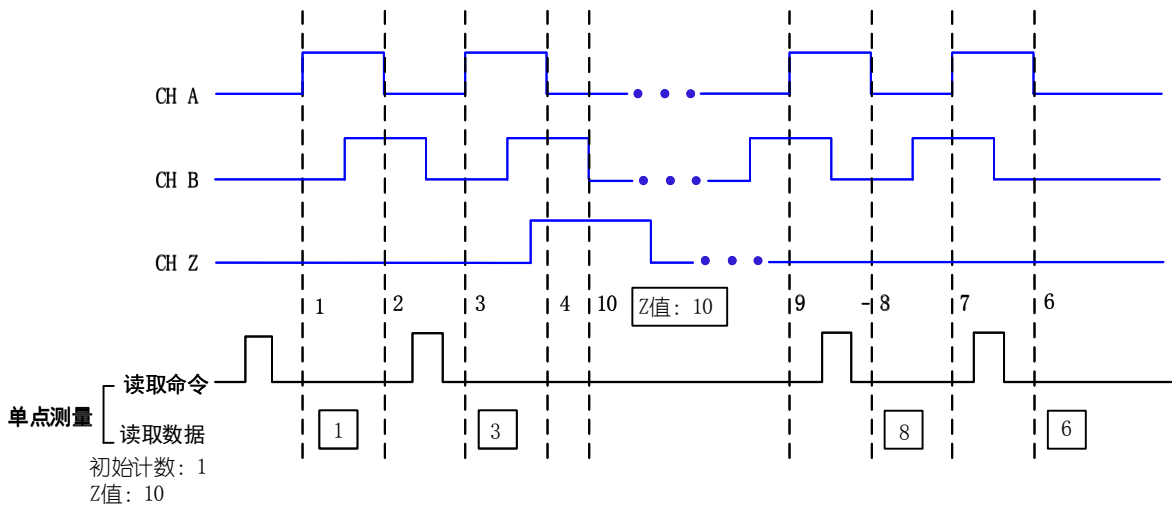
图 6-7-6 Z 索引
