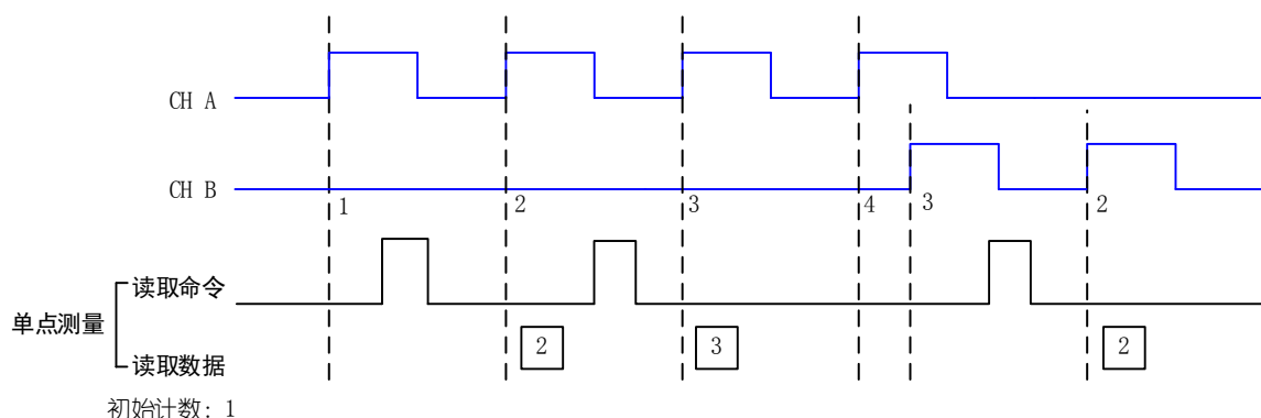
图 6-7-4 双脉冲编码
