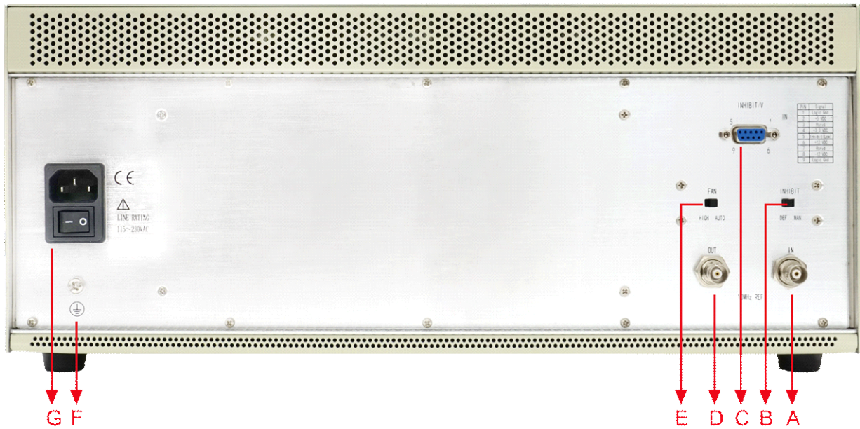
图3 PXIeC-7318C 后面板
