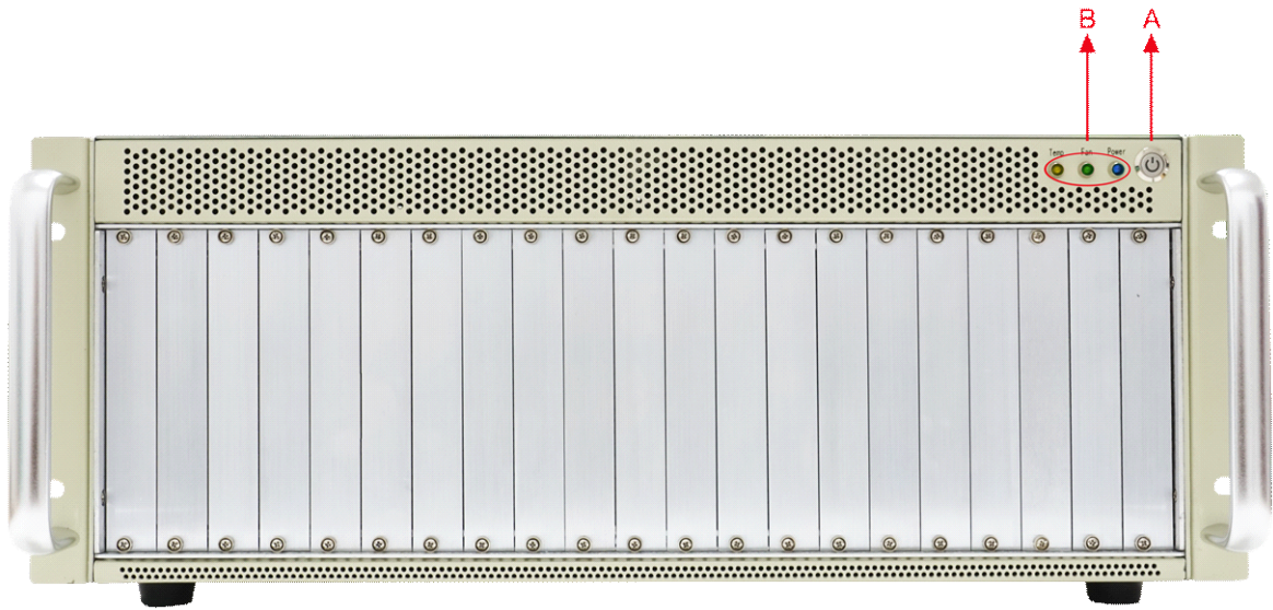
图 1 前面板图
