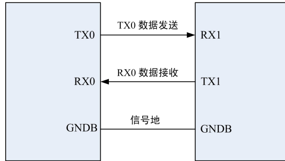
图 4-1-1 三线制信号连接
