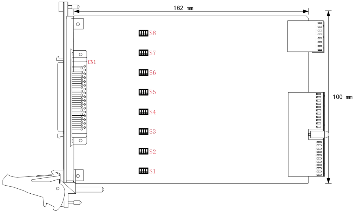
图 1-1-1 PCH6200A 尺寸图
