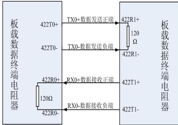
图 4-1-4 RS422 信号连接
