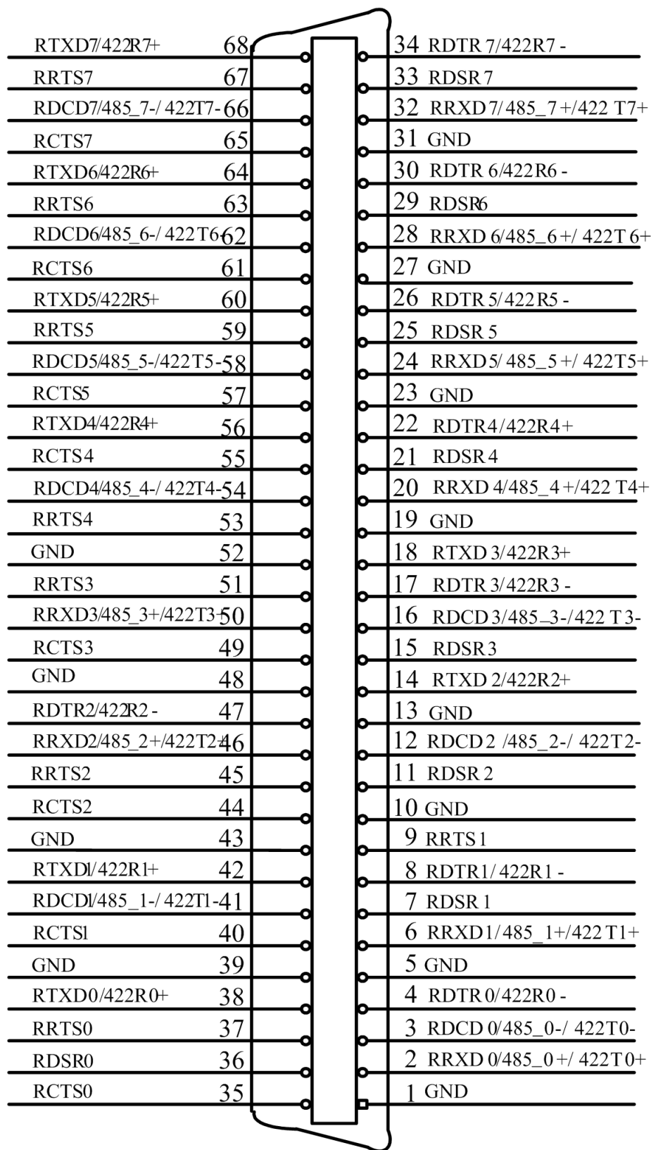
图 3-1-1 P1 的管脚定义
