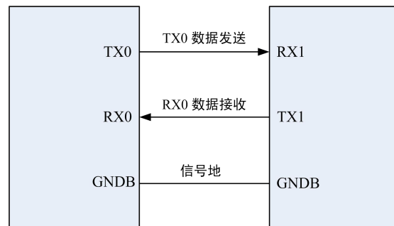
图 4-1-2 全功能串口信号连接
