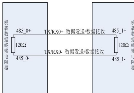
图 4-1-3 RS485 信号连接
