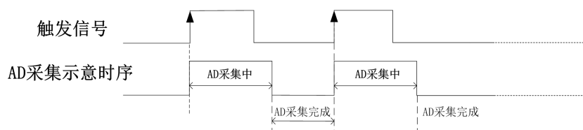
图 4-10-1 触发时序示意图
