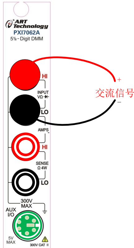
图 3-3-1 测量逻辑频率接线方式
