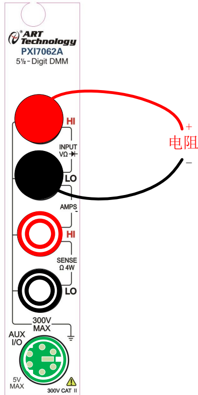
图 3-6-1 2W 电阻测量接线方式
