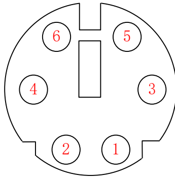
图 2-2-2 J5 引脚定义
