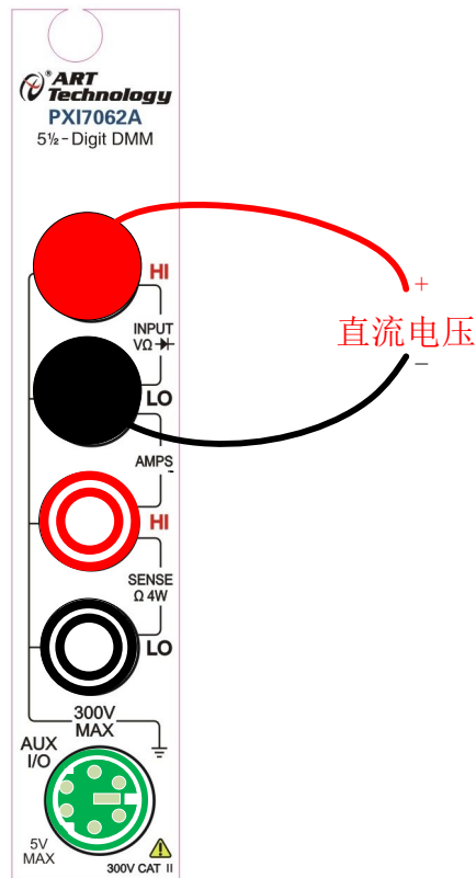
图 3-2-1 测量直流电压接线方式
