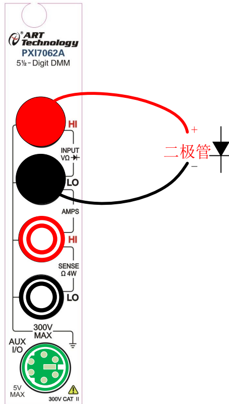
图 3-4-1 二极管测量接线方式
