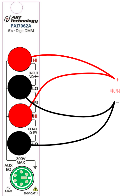
图 3-7-1 4W 电阻测量接线方式
