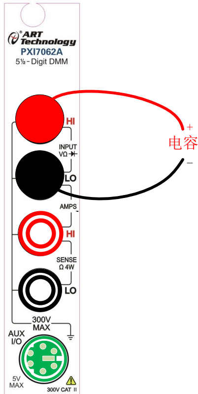
图 3-5-1 测量电容接线方式
