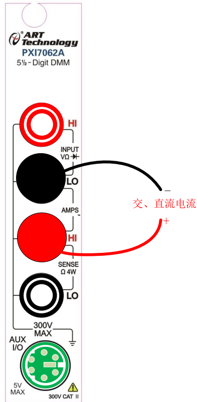
图 3-8-1 测量交、直流电流接线方式
