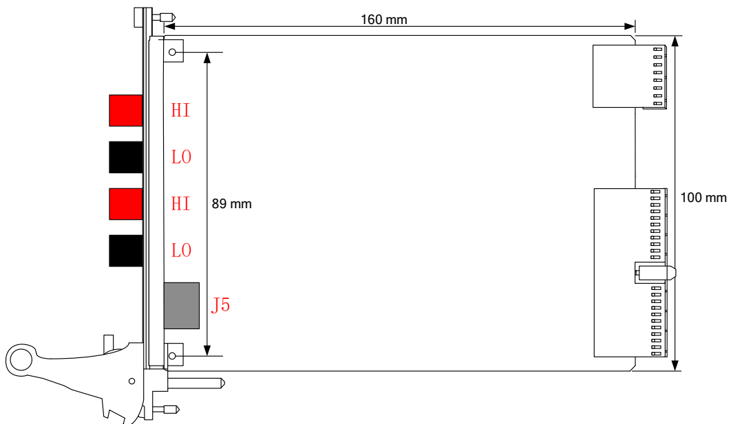
图 2-2-1 板卡尺寸图
