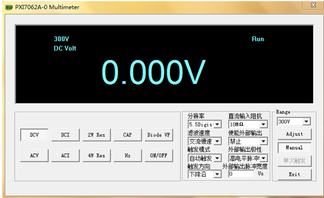
图3-1操作界面图
