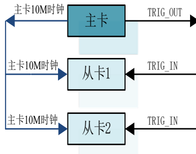
图 4-10-1 主从卡级联
