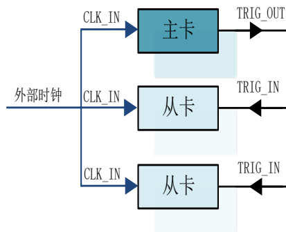
图 4-10-2 采用共同外时钟
