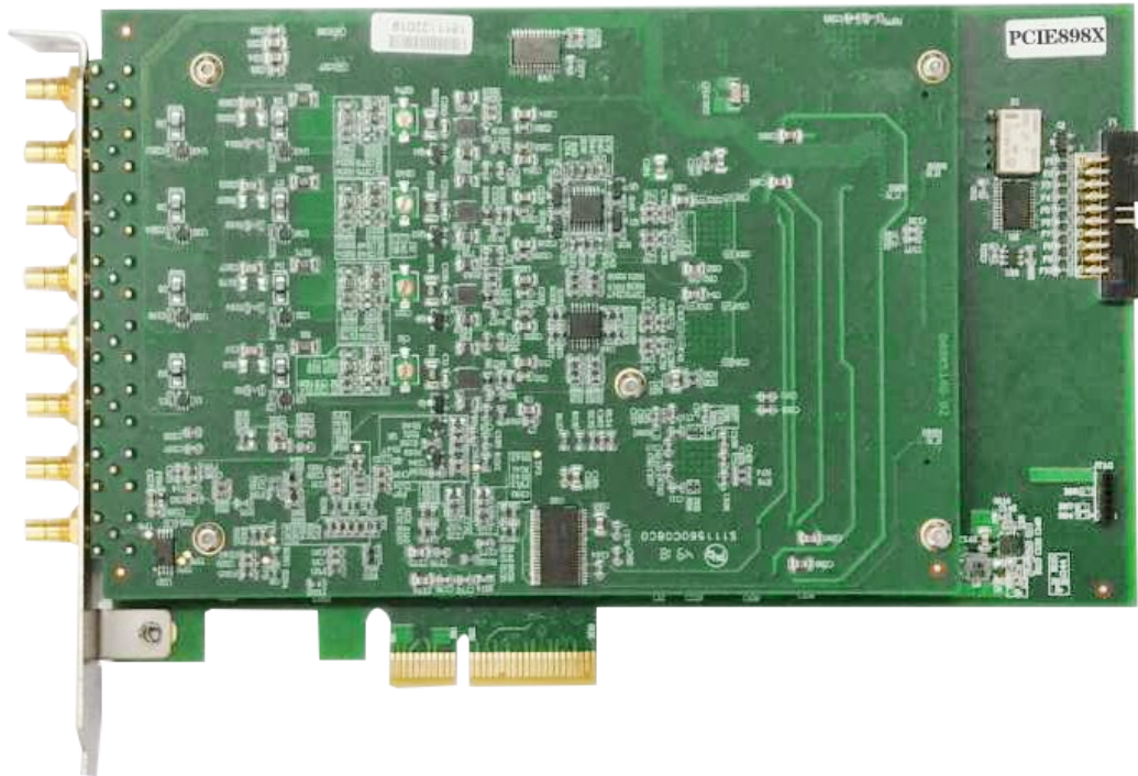
图 3-3-1 PCIe8504/8514 产品外观图
