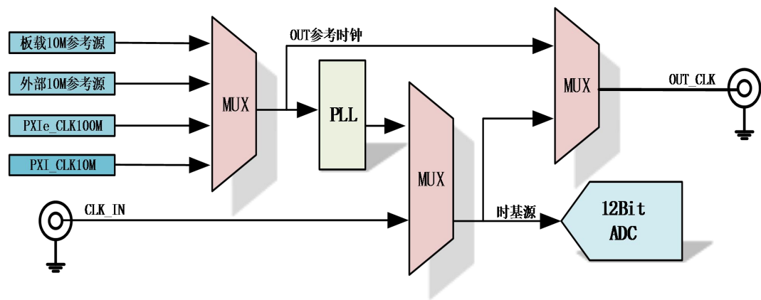
图 4-7-1 时基源框图
