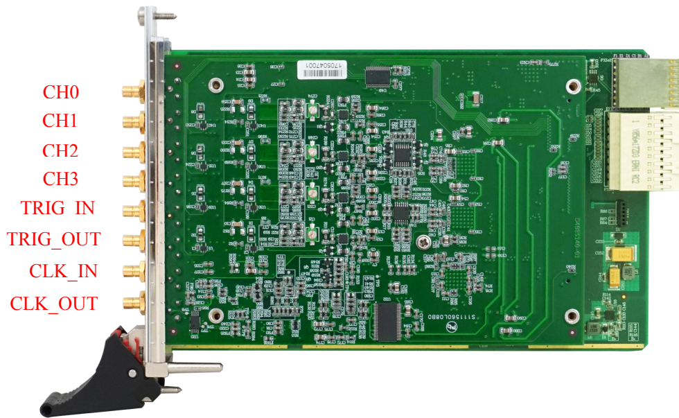
图 3-3-1 PXIe8502/8512 产品外观图
