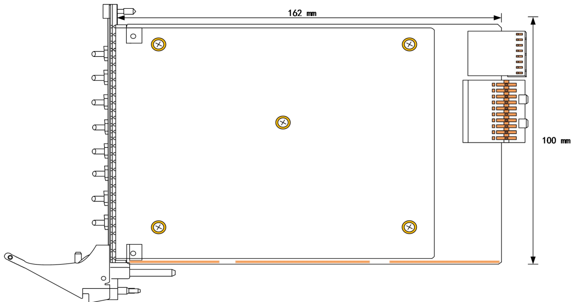
图 3-2-1 PXIe8502\8512 板卡尺寸图
