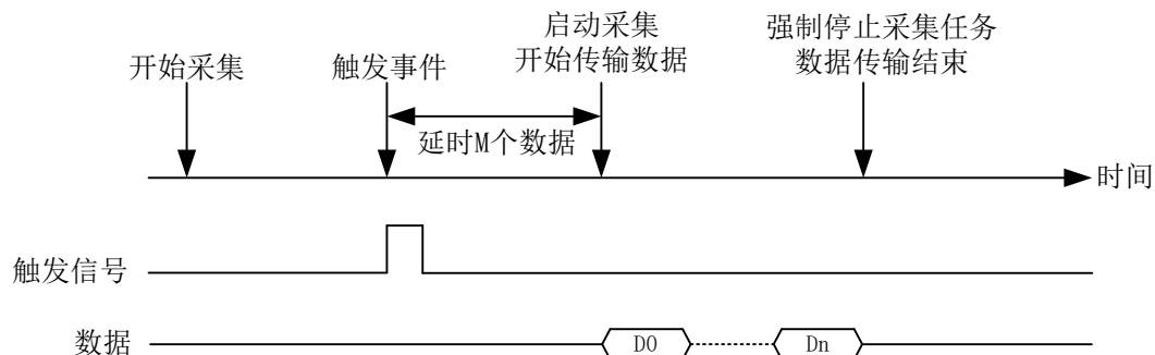
图4-9-1-2 硬件延时触发模式下连续采样
