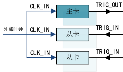
图 4-10-2 共同的外时钟
