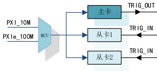
图 4-10-1 采用背板时钟信号作为时钟参考源
