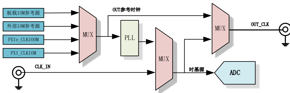
图 4-7-1 时基源框图
