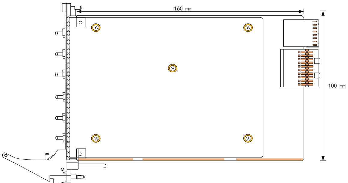
图 3-2-1 PXIe891x 板卡尺寸图
