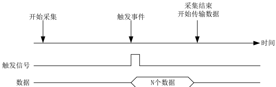
图 4-9-2-3 后触发
