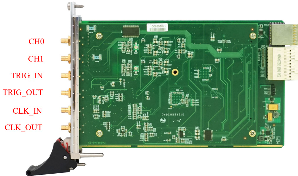
图 3-3-1 PXIe891x 产品外观图
