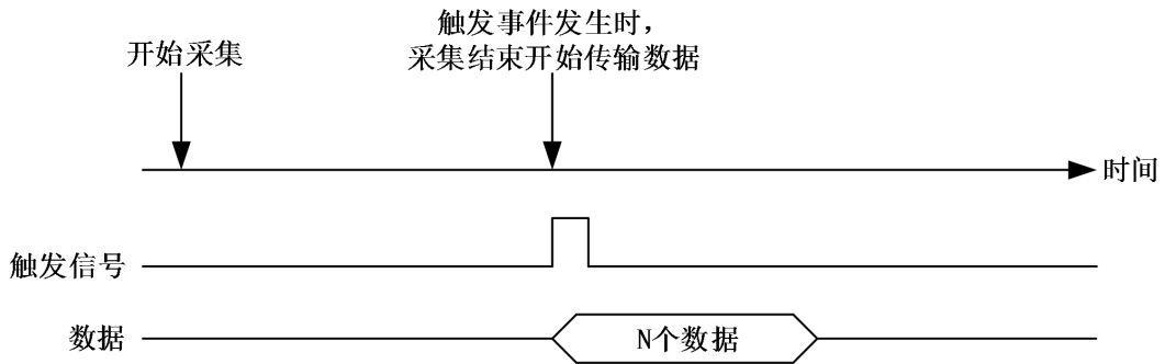
图 4-9-2-3 后触发
