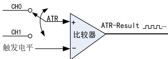
图 4-8-5 比较器
