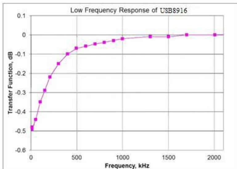
图 4-1-2 USB8916 低频响应
