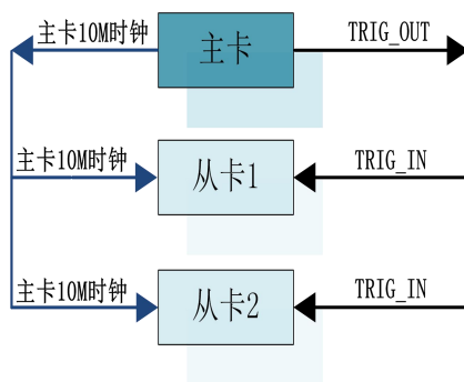
图 4-10-1 主从卡级联
