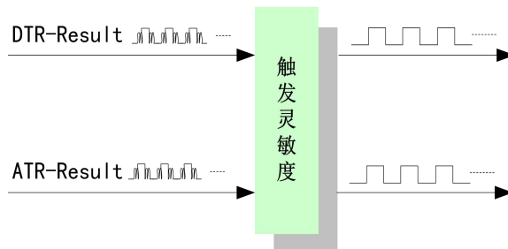
图 4-8-2 触发灵敏度
