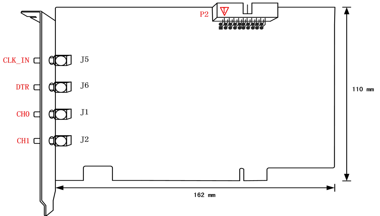
图 3-2-1 PCI-8552B/8554B 板卡尺寸图
