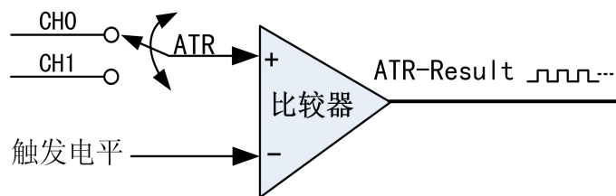
图 4-9-5 比较器
