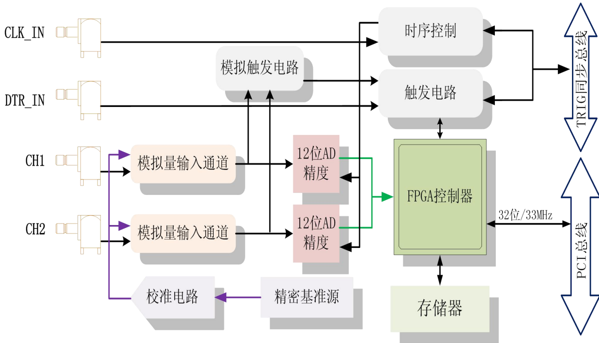
图 3-1-1 PCI8552B 系统框图
