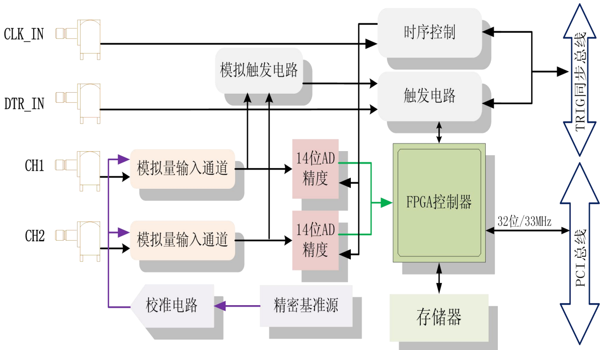
图 3-1-2 PCI8554B 系统框图
