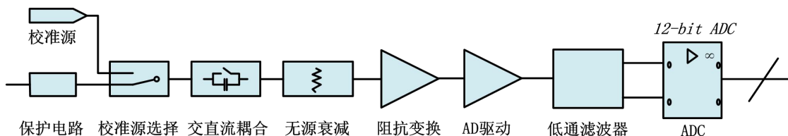
图 4-1-1 PCI8552BAD 功能框图
