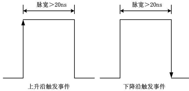
图 4-9-8 脉宽最小值图
