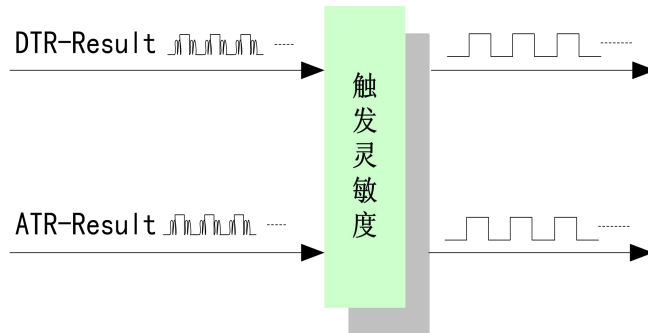
图 4-9-2 触发灵敏度
