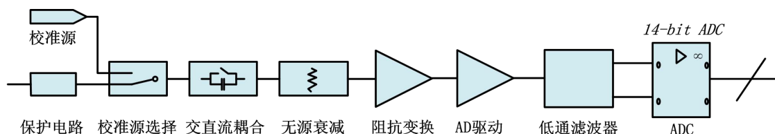
图 4-1-2 PCI8554BAD 功能框图
