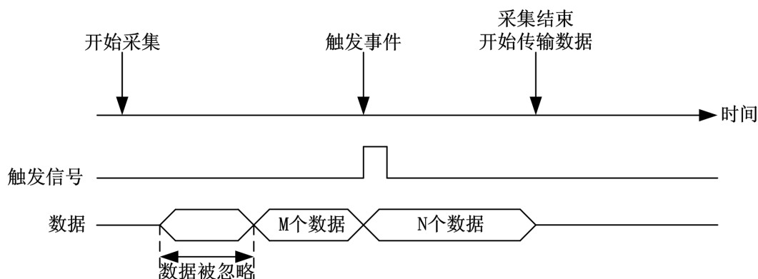
图 4-10-2 中间触发
