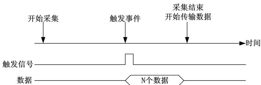
图 4-10-3 后触发
