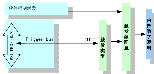
图 4-9-1 AI 触发功能框图
