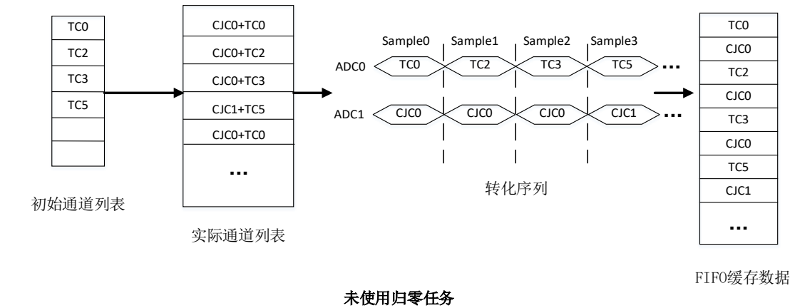
图 4-4-1 不启动归零
