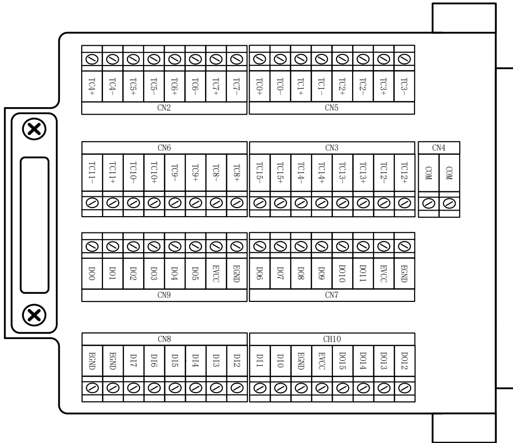
图 3-3-1 TB8091 端子引脚定义
