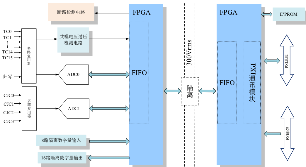
图 2-2-1 PXI8091 系统框图
