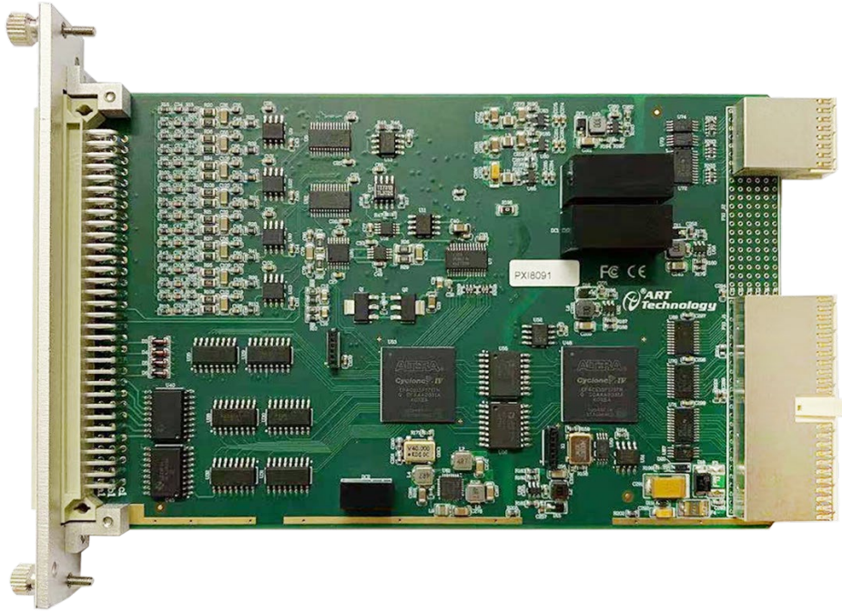
图 3-1-1 PXI8091 外形图
