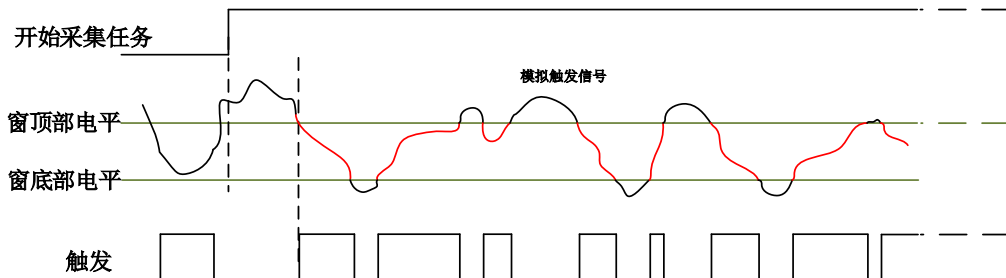
图4-8-8 模拟窗触发--入窗
