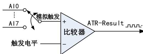
图4-8-5 比较器
