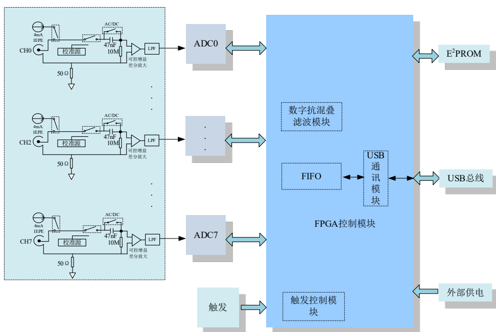
图 2.2.1 USB8814 系统框图
