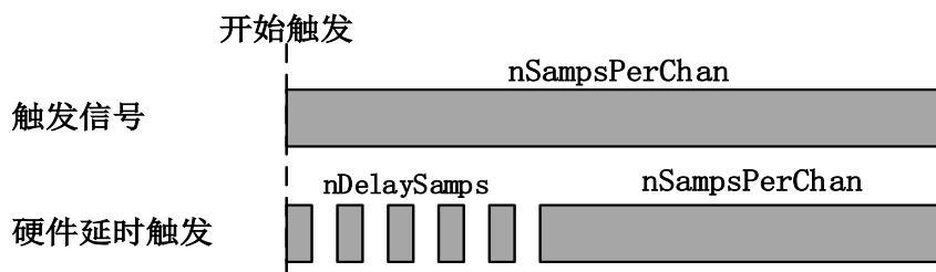
图 4-7-1 AI 触发模式
