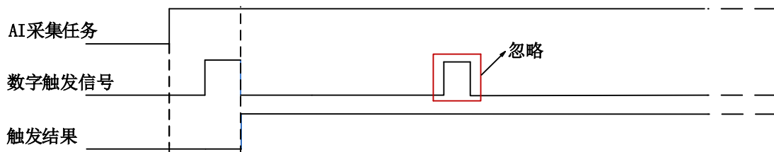
图4-8-10 数字边沿触发--下降沿触发
