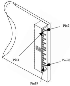
图 3-2-2 RTSI 的 Pinout 图
