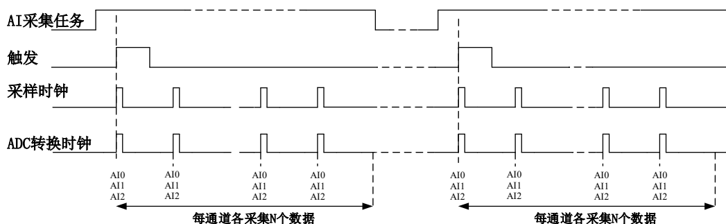
图4-6-2 有限点采样
