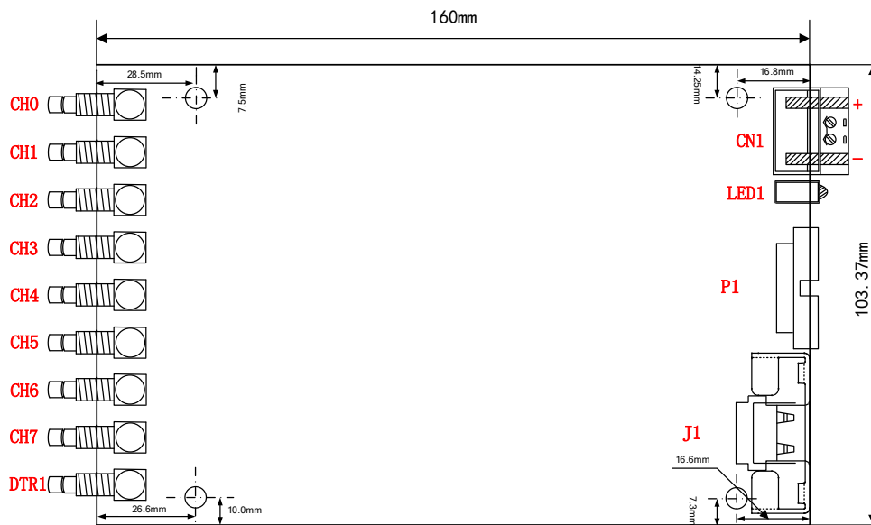
图 3-2-1 板卡尺寸图
