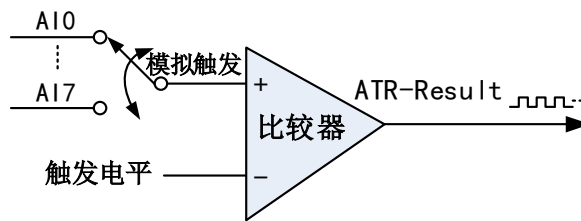
图4-8-7 比较器
