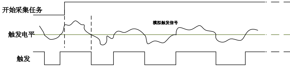
图4-8-6 模拟边沿触发--下降沿触发
