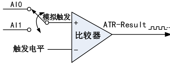
图6-2-7 比较器
