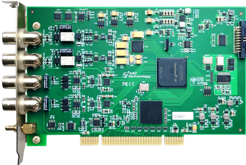
图 3-1-1 PCI8822 外形图（图片仅供参考）
