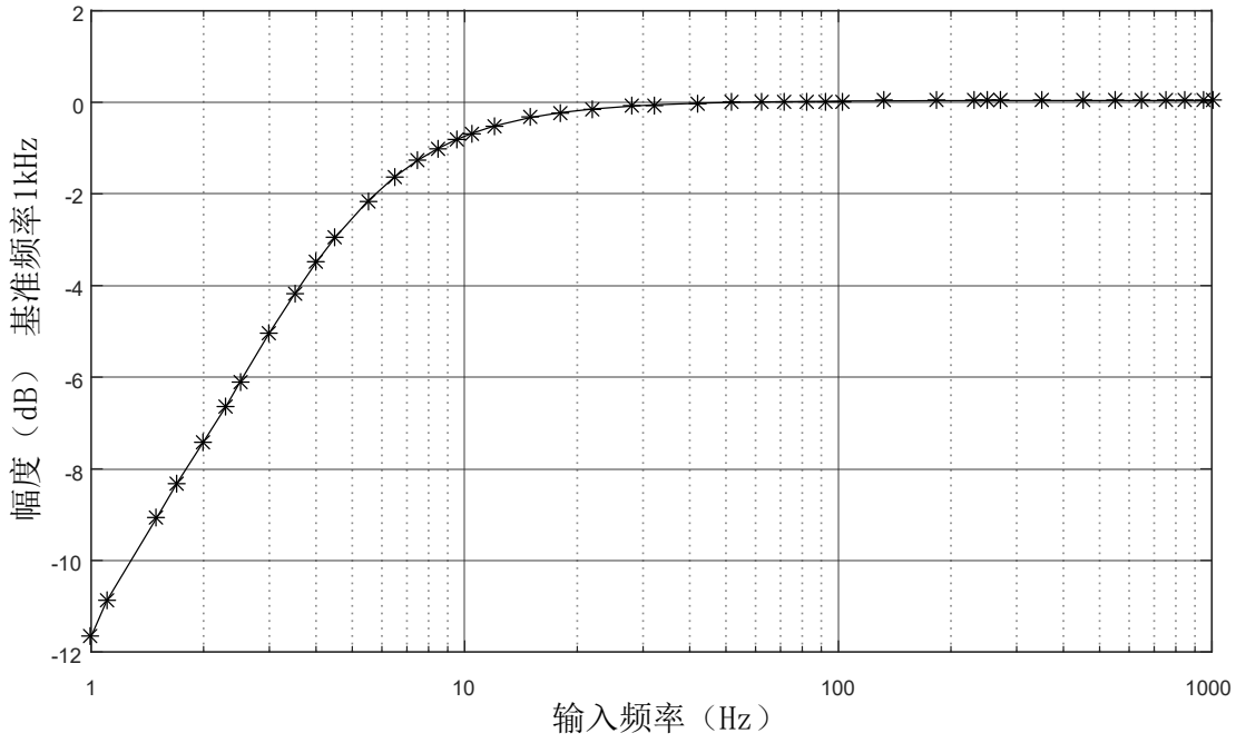
图 2-2-1 交流耦合电路的幅度响应(1Hz~1kHz)
