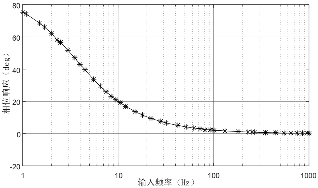
图 2-2-2 交流耦合电路的相位响应(1Hz~1kHz)
