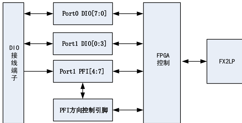
图7-1-1 DIO功能框图
