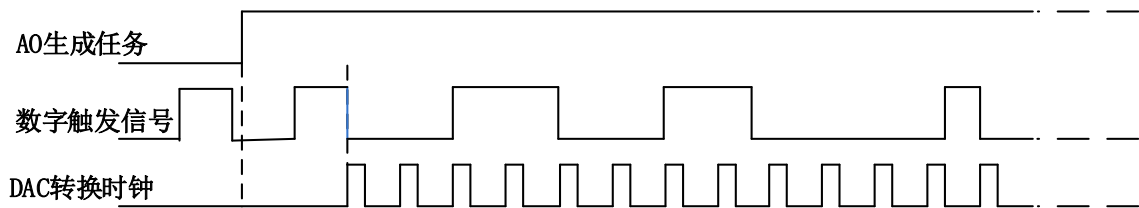
图 5-8-5 数字触发--下降沿触发
