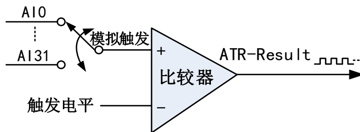
图4-9-5 比较器
