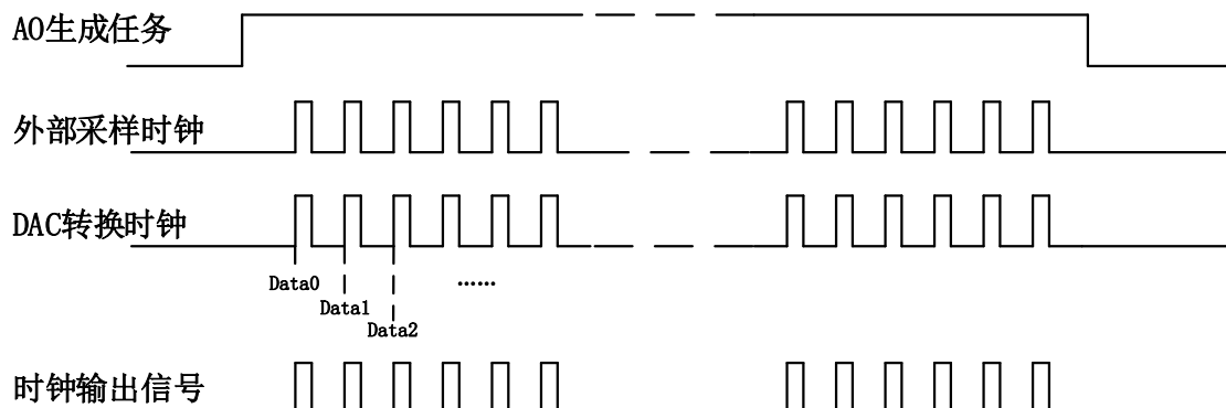
图 5-6-3 外时钟时序图
