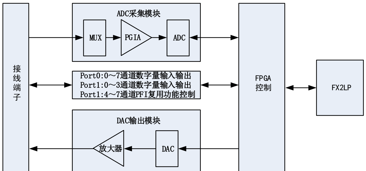
图2-2-1 USB3120/21/22系统框图
