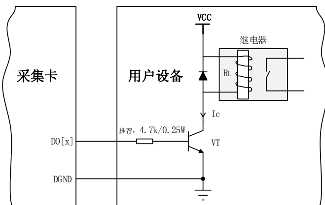
图 7-3-3 DO 数字量控制继电器电路
