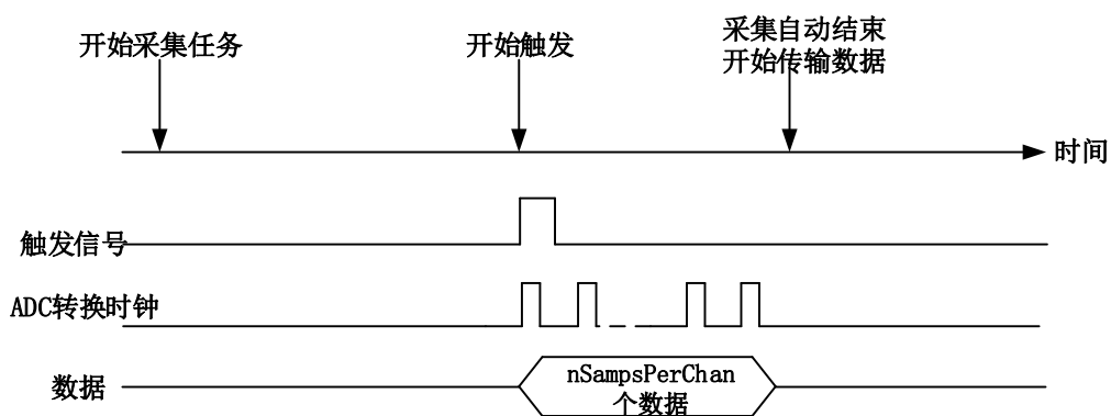
图 4-10-2 开始触发
