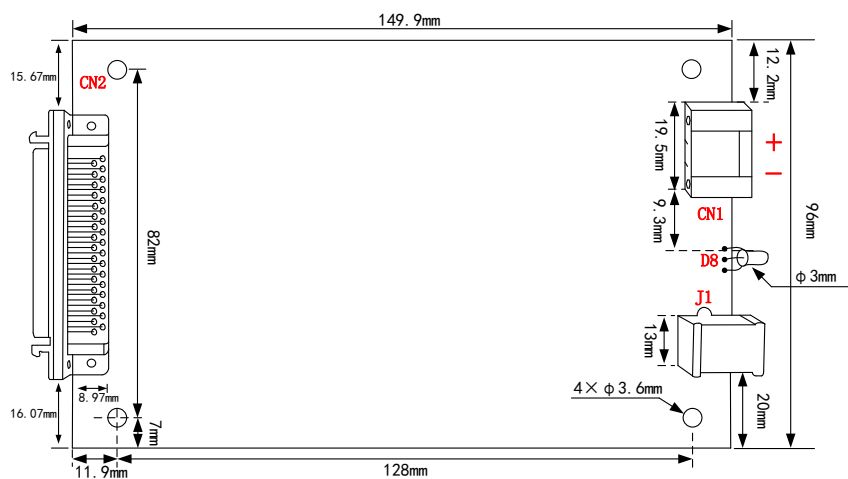
图 3-2-1 板卡尺寸图
