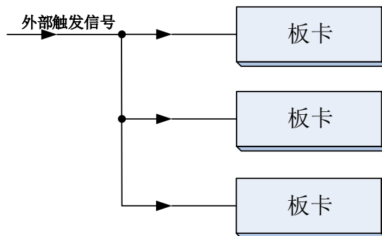
图 4-11-2 外触发同步采集的连接方式
