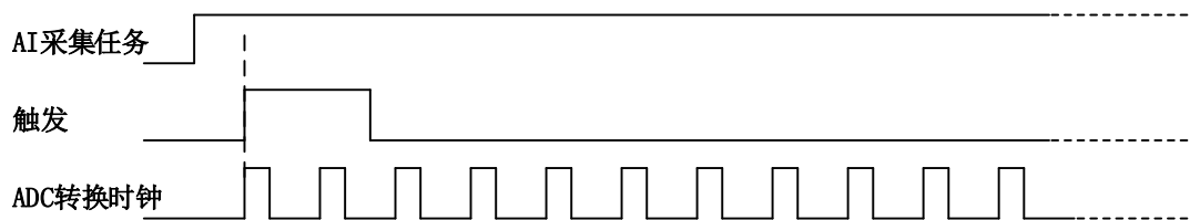
图4-9-3 AI软件强制触发
