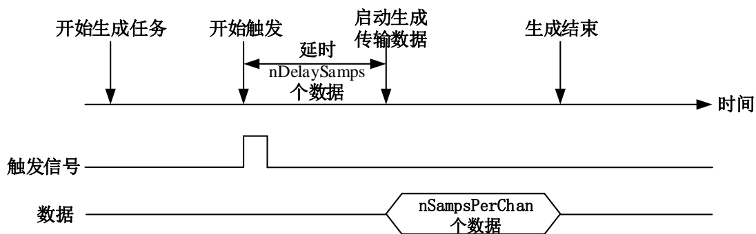
图 5-9-1 延时触发
