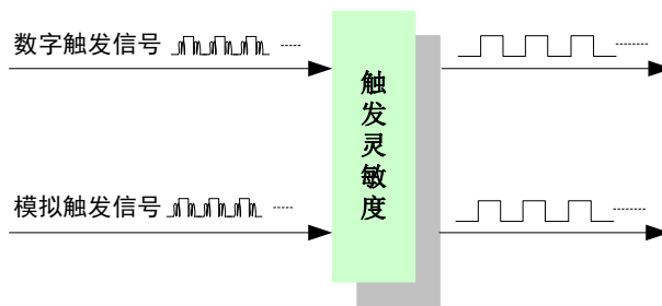
图 4-9-2 触发灵敏度
