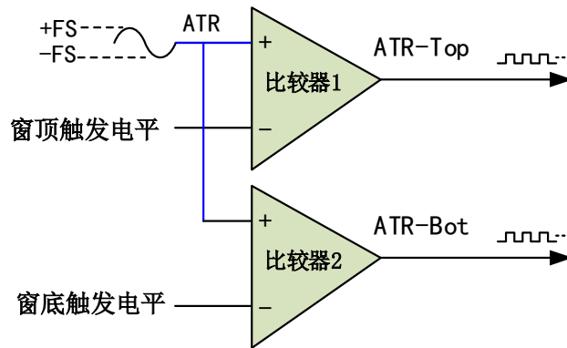
图7-3-6 比较器
