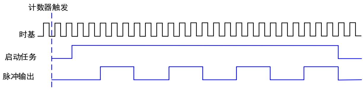
图 5-8-3 有限脉冲序列生成
