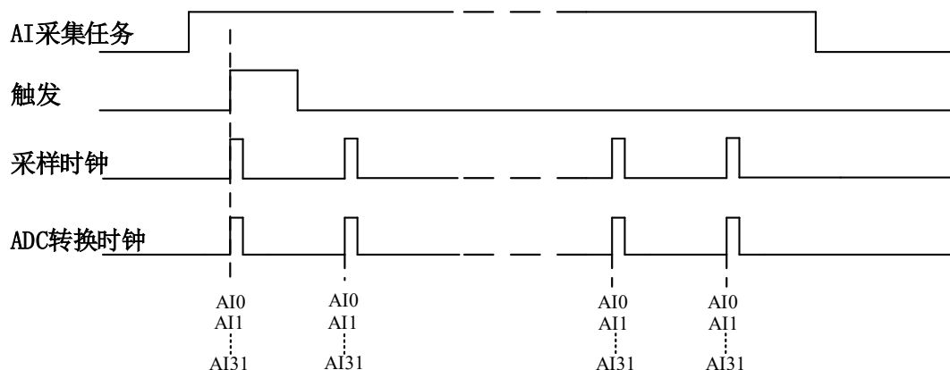
图4-7-3 时钟连续采样
