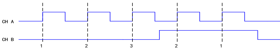
图 5-7-5 单脉冲编码
