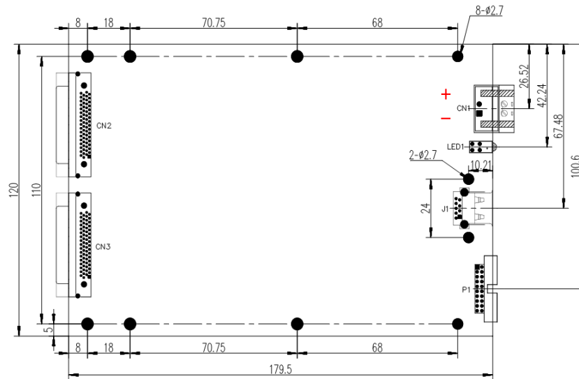
图 3-2-3 板卡尺寸图
