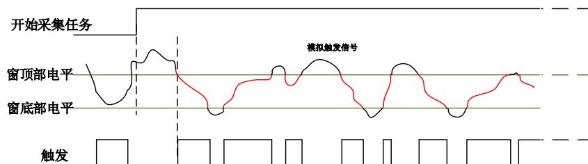
图7-3-7 模拟窗触发--入窗
