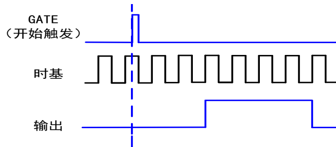
图 5-8-2 具有开始触发的单脉冲生成
