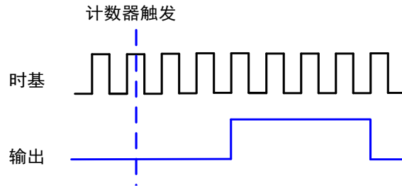
图 5-8-1 单脉冲生成
