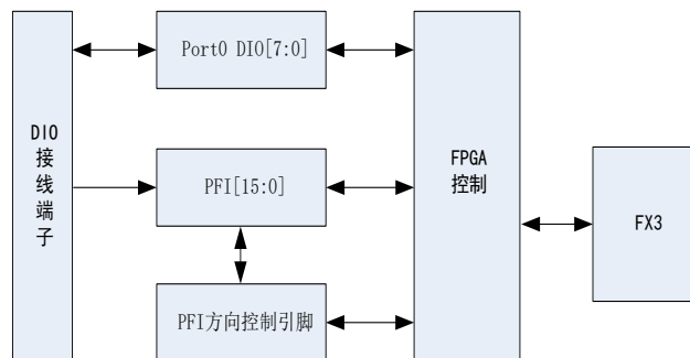
图6-1-1 DIO功能框图
