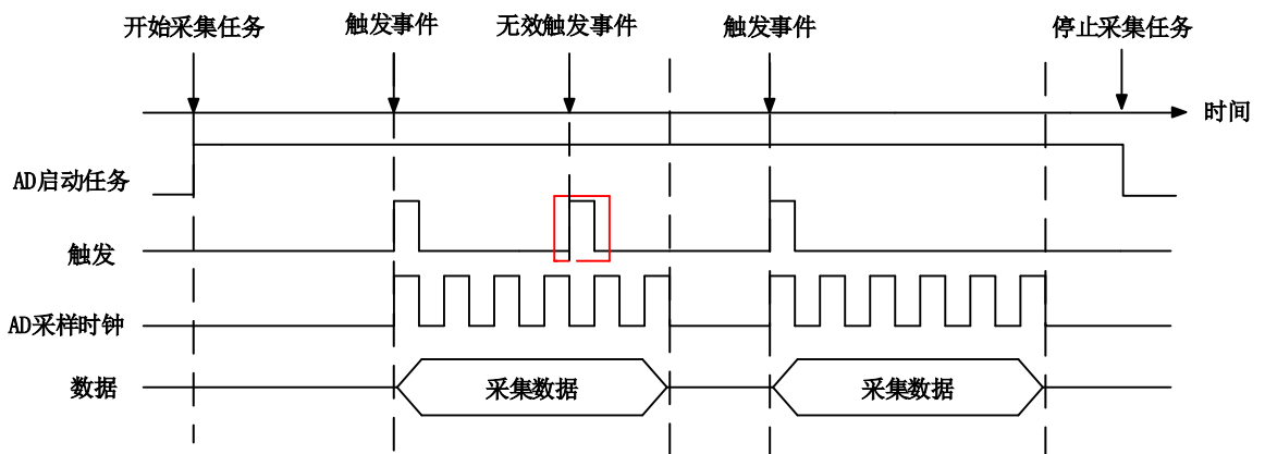
图 7-2-6 重触发
