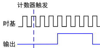
图 5-8-1 单脉冲生成
