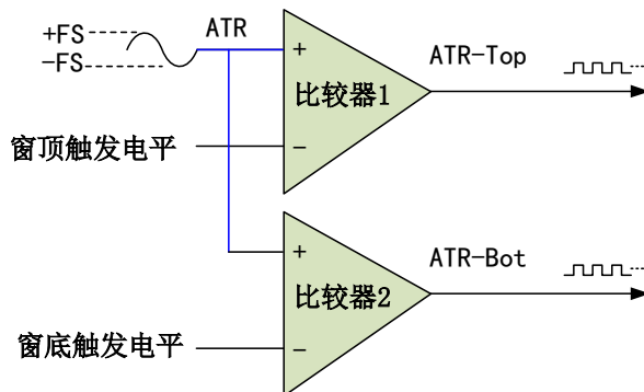
图7-3-6 比较器
