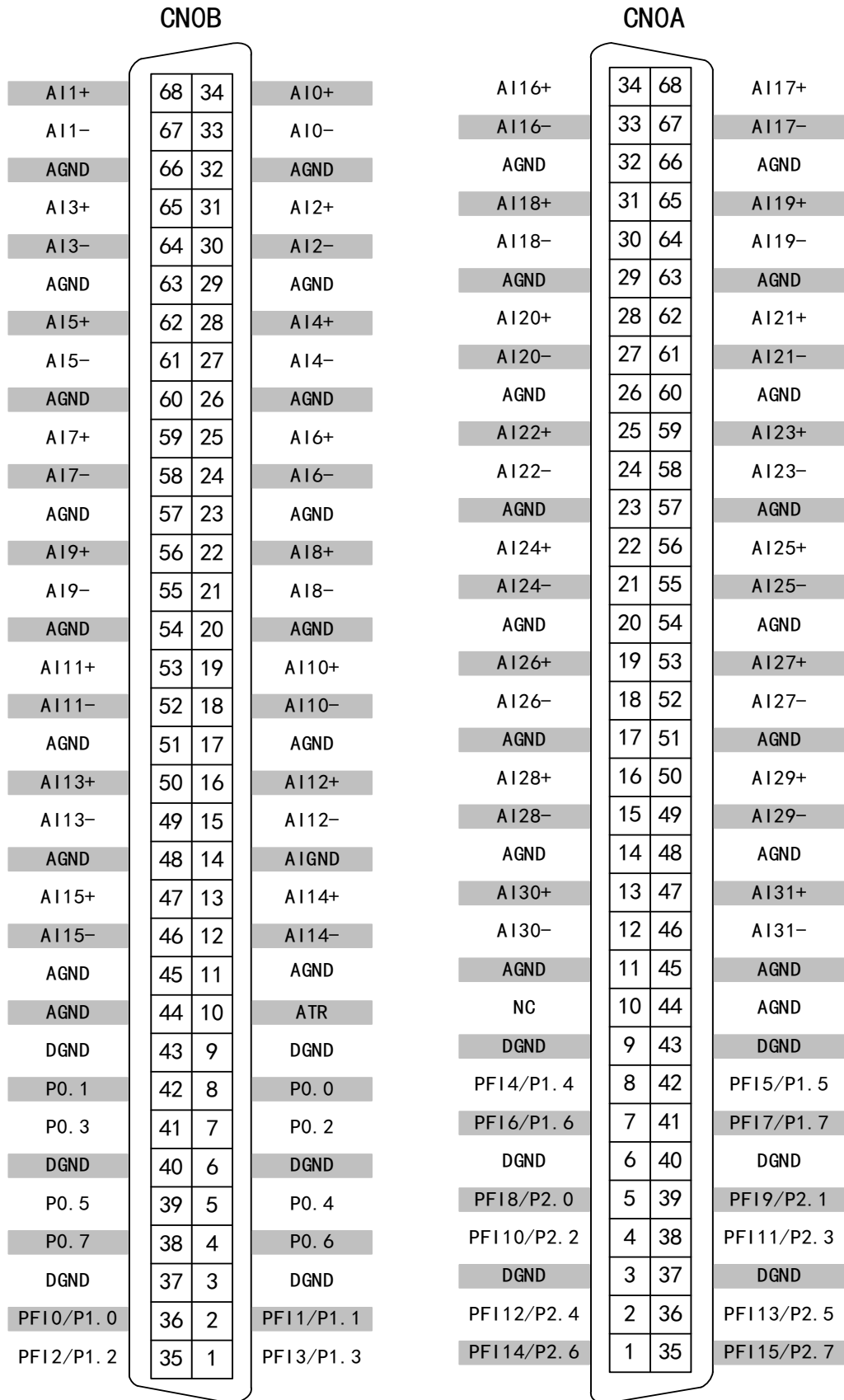
图3-3-1 管脚定义
