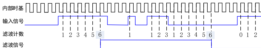
图 5-9-1 数字滤波
