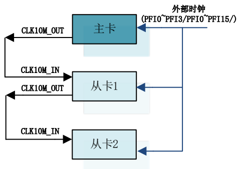
图 4-9-2 共同外时钟
