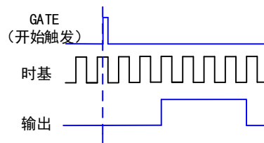
图 5-8-2 具有启动触发的单脉冲生成
