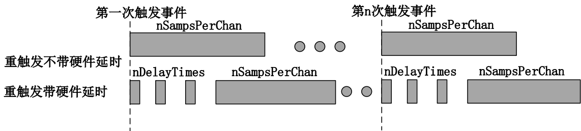
图7-2-5 AI重触发
