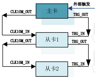
图 4-9-1 共同外部触发信号
