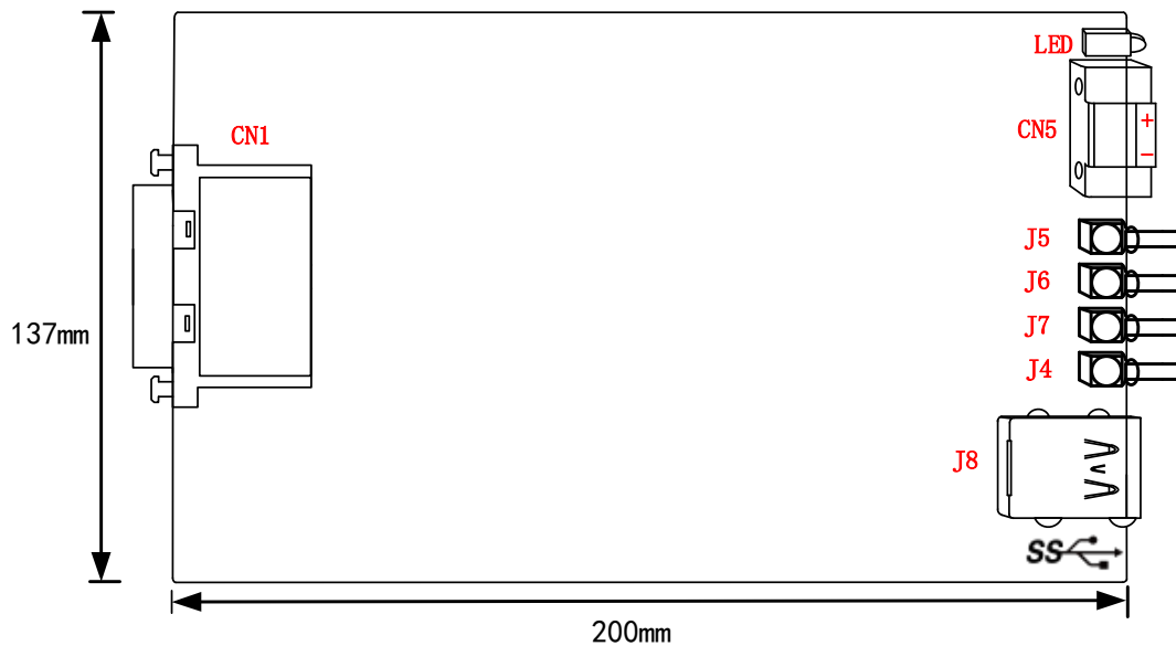
图 3-2-1 板卡尺寸图
