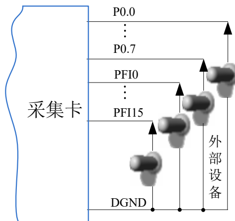
图6-2-1 DI 数字量输入的连接
