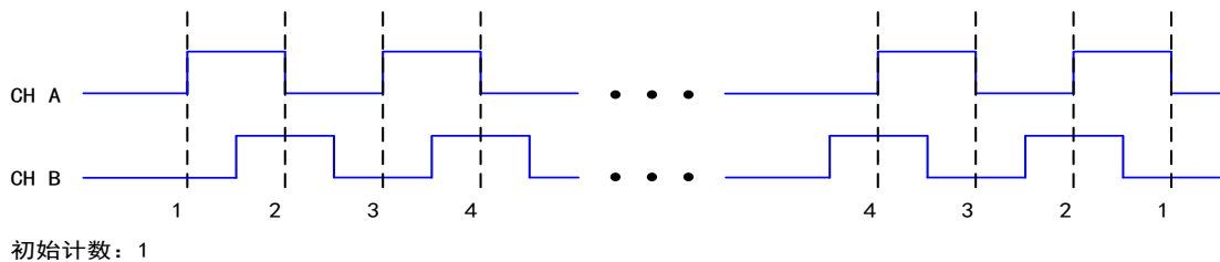
图 5-7-2 X2 编码
