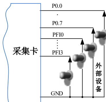
图6-2-1 DI 数字量输入的连接
