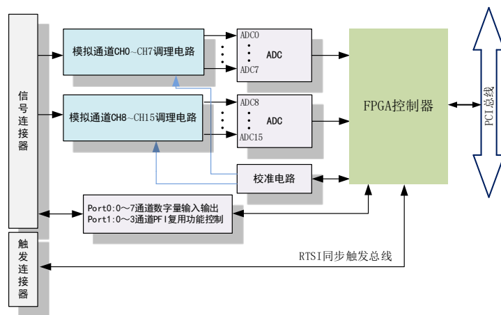
图 2-2-1 PCI9009/A/B 系统框图
