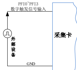
图7-3-8 数字触发连接方法
