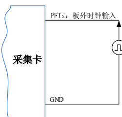
图 6-4-1 时钟输入输出的连接
