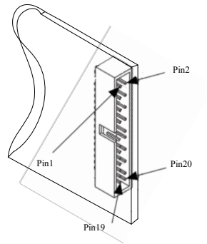
图 3-3-2 RTSI 的 Pinout 图
