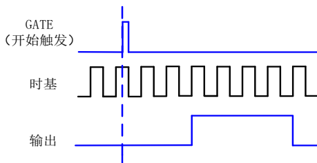
图 5-8-2 具有启动触发的单脉冲生成
