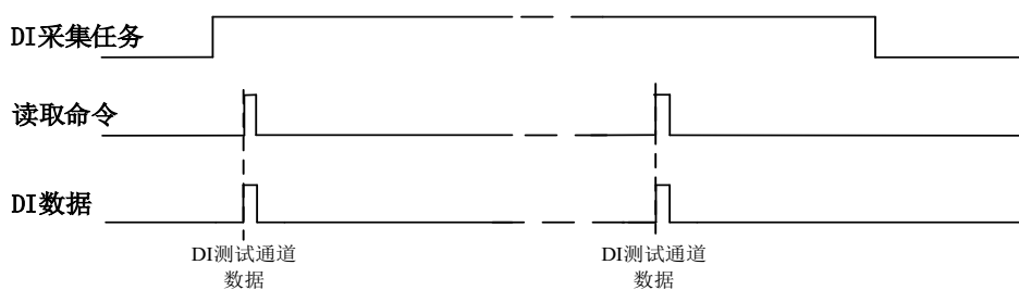
图7-6-1 按需单点采集
