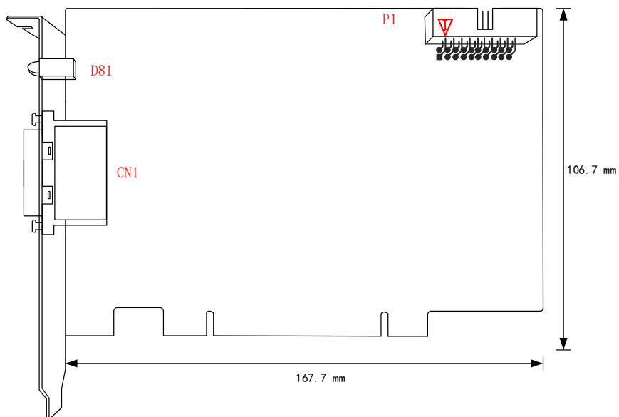
图 3-2-1 PCI9774 板卡尺寸图
