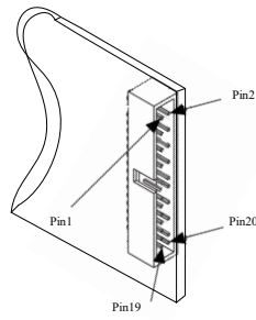
图 3-3-3 RTSI 的 Pinout 图
