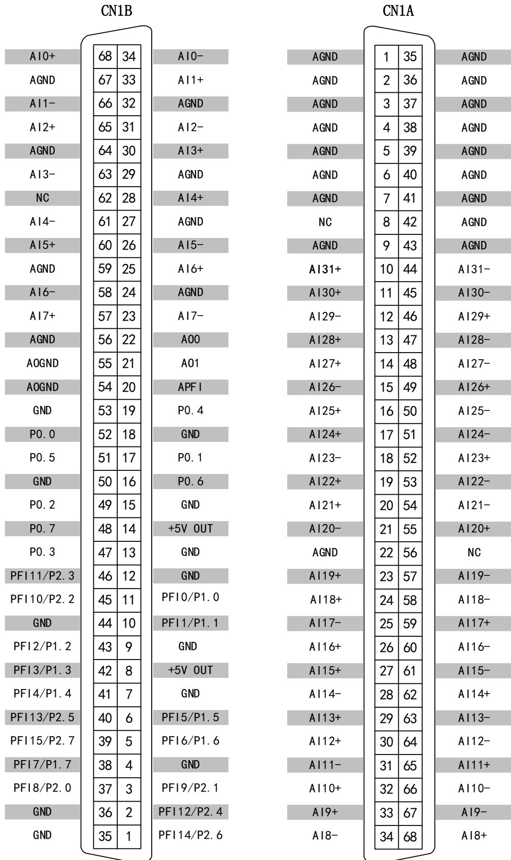
图3-3-2 PCI9774 CN1连接器管脚定义
