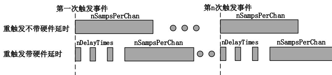
图 8-2-4 重触发
