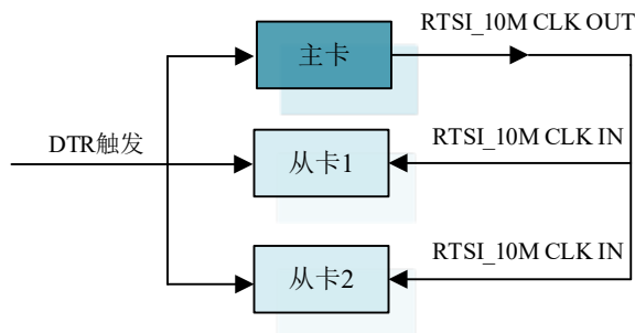
图 4-9-1 采用 RTSI_10M 时钟主从卡同步的级联方式（推荐）
