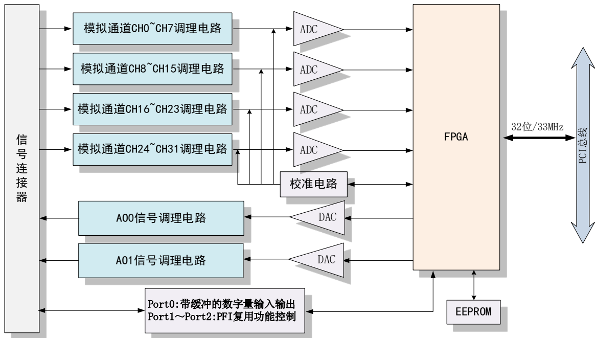
图2-2-1 PCI9774系统框图
