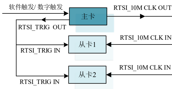
图 4-9-2 采用 RTSI_TRIG 触发主从卡同步的级联方式
