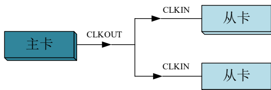
图 4-9-3 主从卡时钟级联同步采集的级联方式
