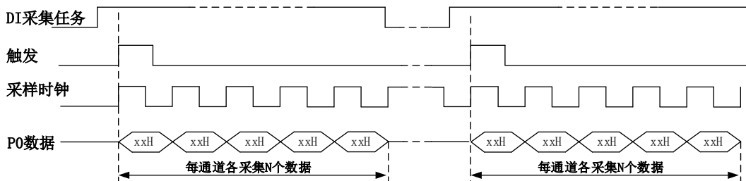
图 5-5-2 有限点采样
