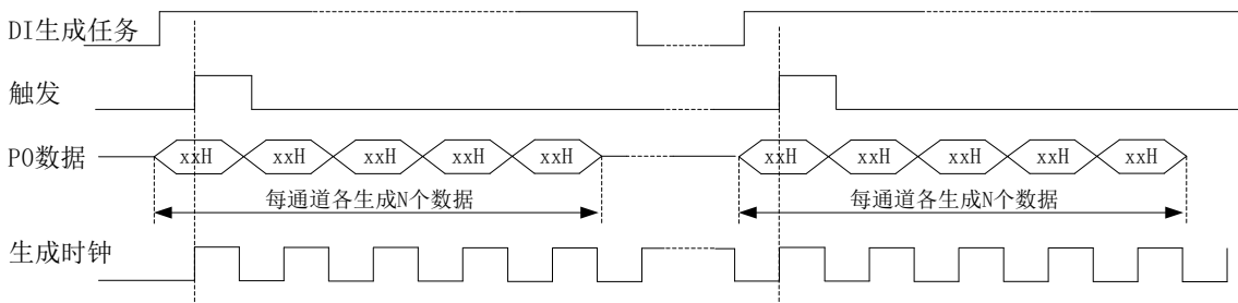
图5-6-2 有限点生成
