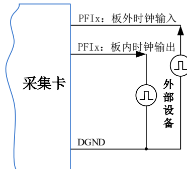
图 5-4-1 时钟输入输出的连接
