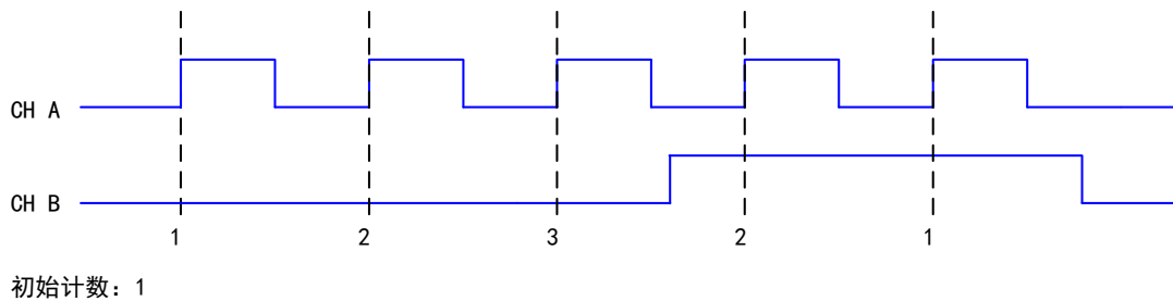
图 6-7-5 单脉冲编码
