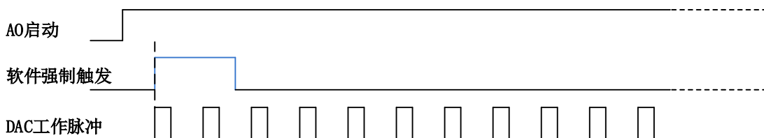
图4-7-4 AO软件触发
