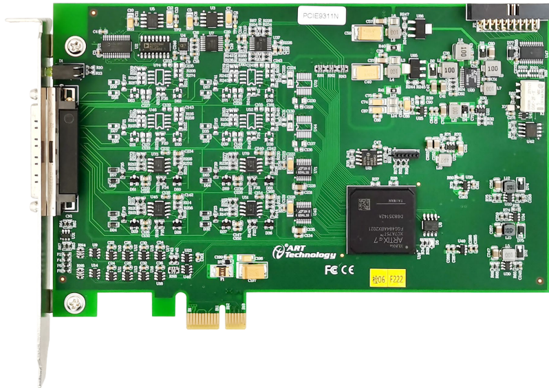
图 3-1-1 PCIe9311N
