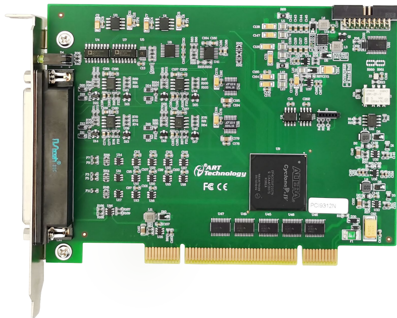
图 3-1-2 PCI9312N
