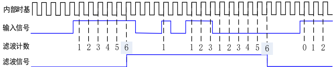
图 6-9-1 数字滤波
